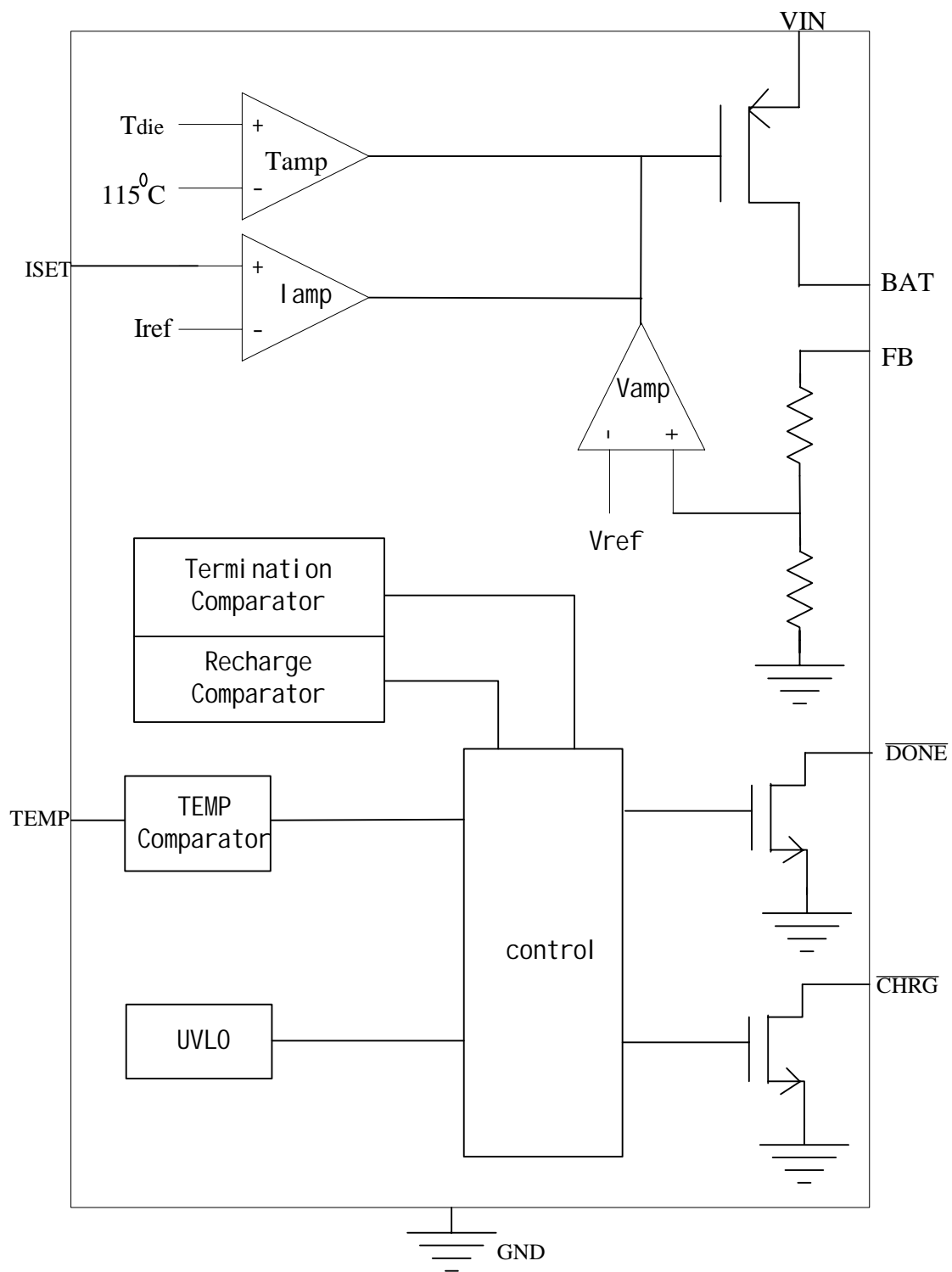
图 3 功能框图
