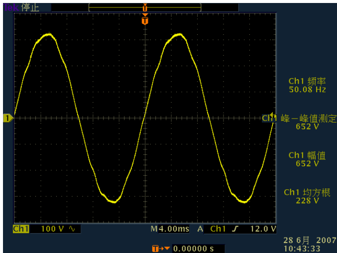
Burn in room 試機區 B20#AC 座 6-2 AC 波形，直流觸發
