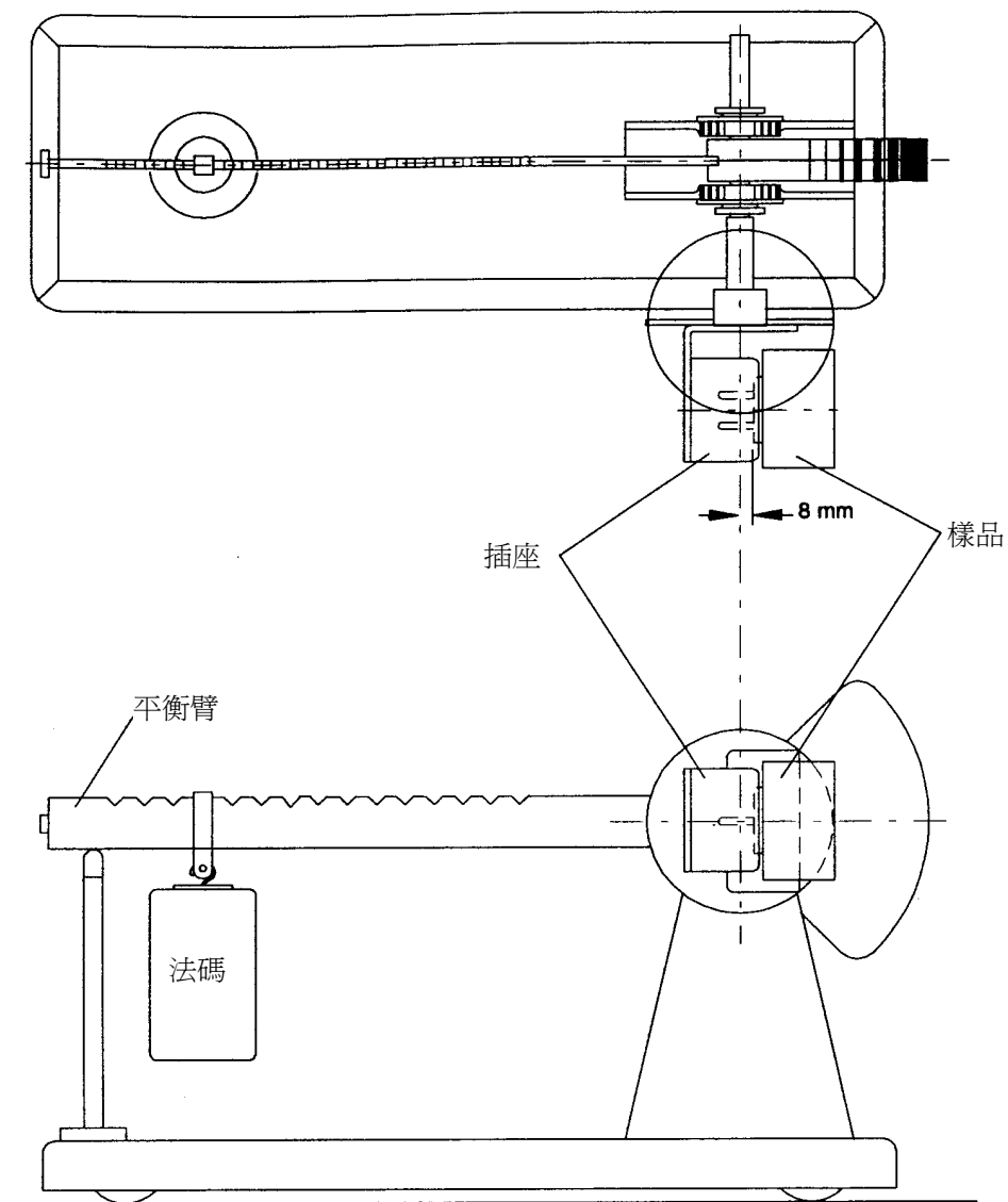
圖 11 電源插頭與設備一體成型之試驗設備
