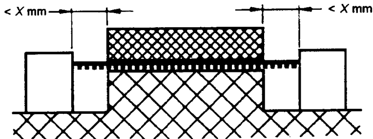
圖 E.6 具寬溝之未強固接合物
