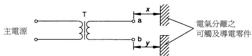
圖 2 強化絕緣之評估
