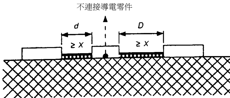
圖 E.9 狹凹
