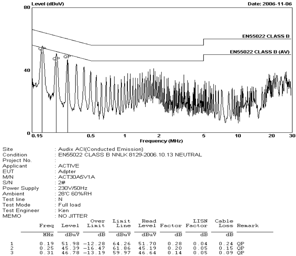
图 12, 传导 EMI, 零线
