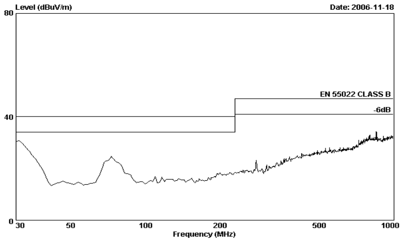
图 13, 辐射 EMI, 垂直
