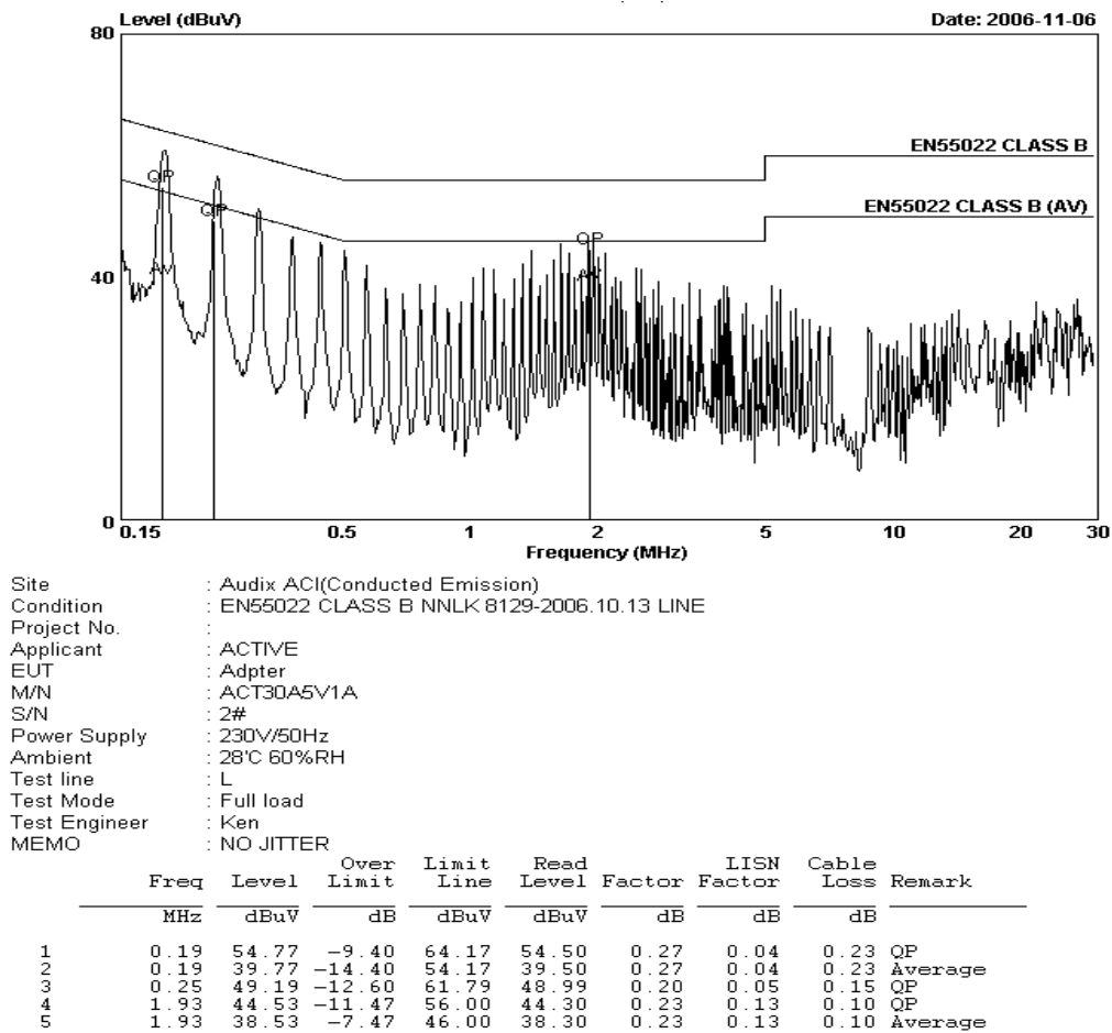
图 11, 传导 EMI, 火线
