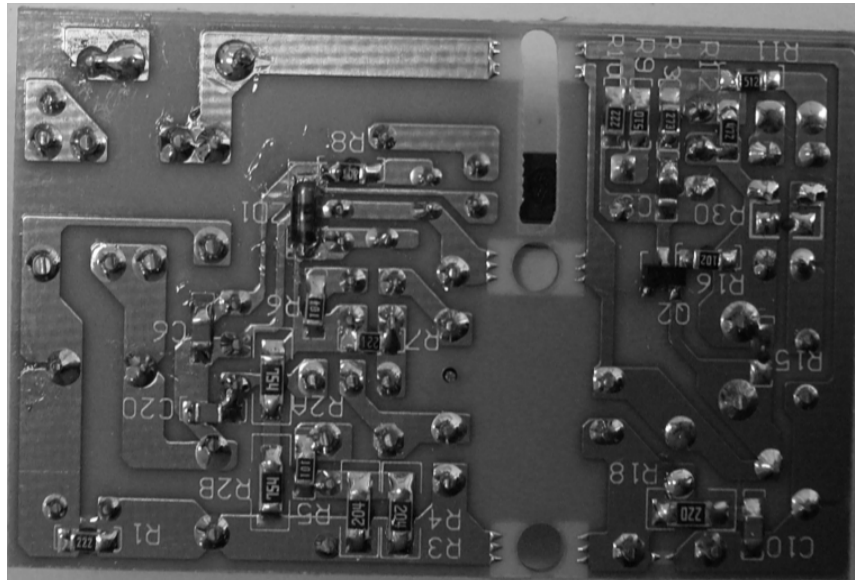
图 2, 背面(68mm x 35mm x 22mm)
