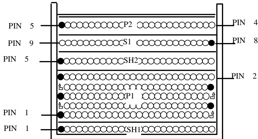
图 6, 变压器装配图
