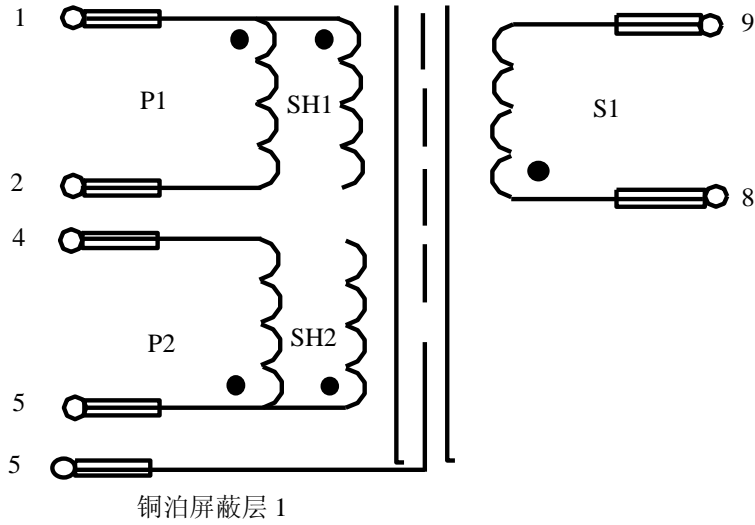
图 5, 变压器示意图
