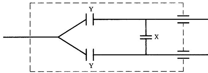
图 5b 三角形连接旁路电容器
