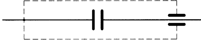
图 5a 单线连接旁路电容器
