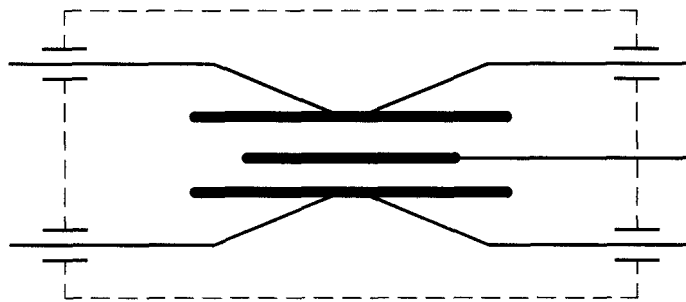
图 4d 多单元穿心电容器
