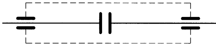
图 1 两个引出端电容器
