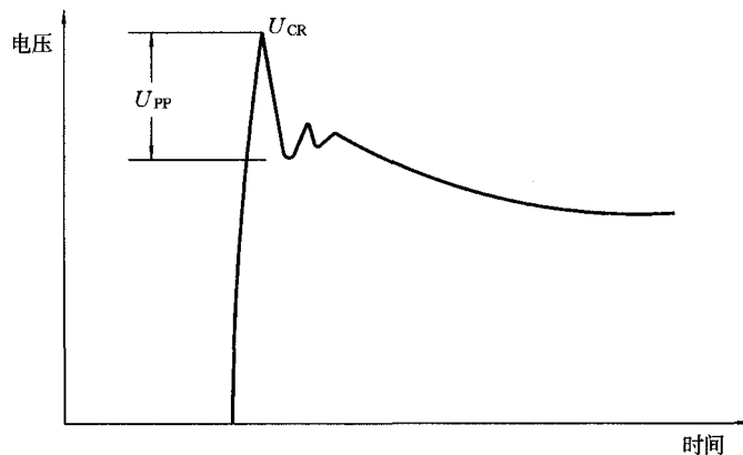
图 6 脉冲波形
