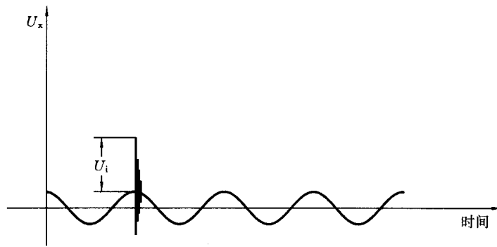
图 8 已叠加随机的非同步高压脉冲的基波交流波形
