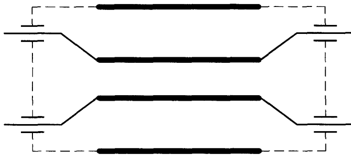
图 4c 对称和非对称使用的多单元穿心电容器(非同轴式)
