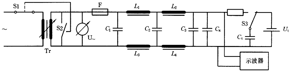
图 7 电容器承受交流电压脉冲典型电路
