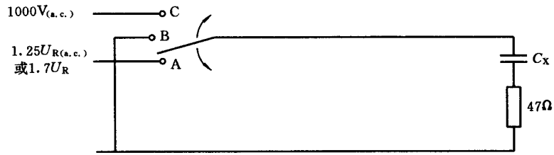
图 B1 耐久性试验电路
