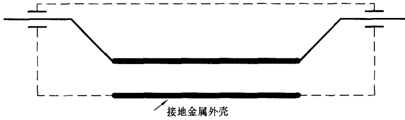
图 4b 非对称使用的穿心电容器(非同轴式)
