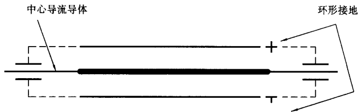
图 3 穿心电容器(同轴式)
