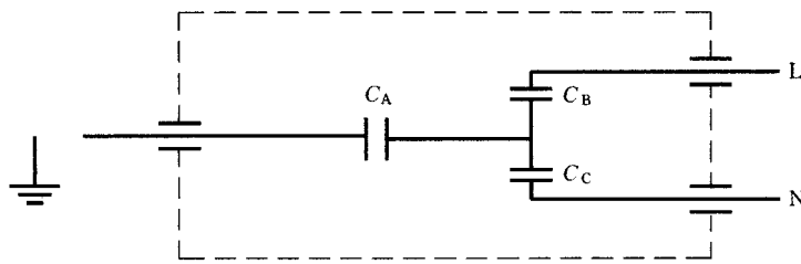
图 5c T形连接旁路电容器
