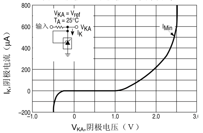
图 5. 阴极电流和阴极电压关系曲线
