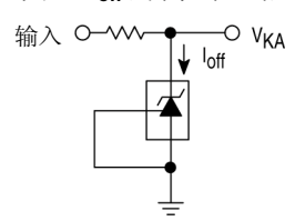
图 3. I_{off} 的测试电路
