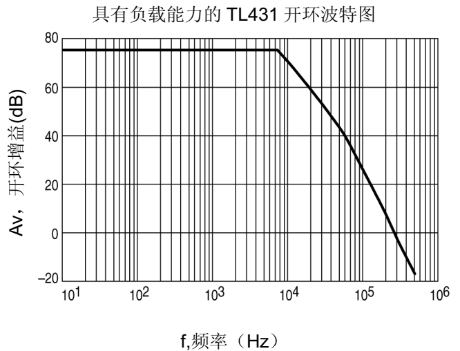
图 33.例 2 电路开环增益图
