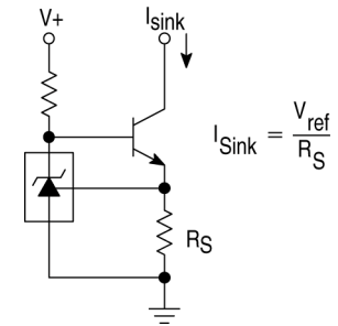
图 23. 恒流宿
