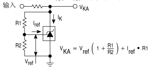
图 2. V_{KA}>V_{ref} 的测试电路
