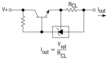
图 22. 恒流源
