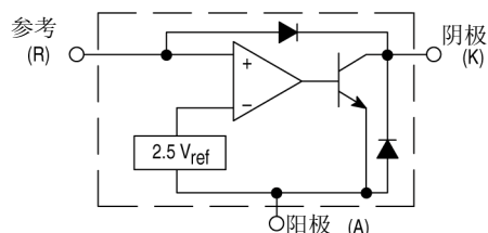
代表性框图
