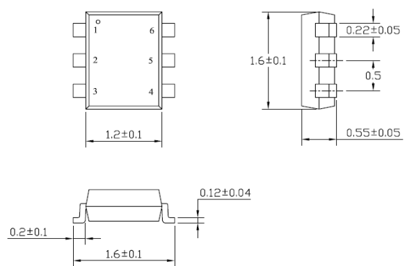
SOT-563
