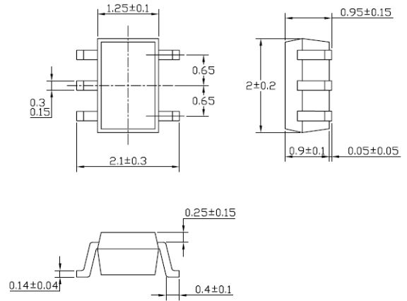
SOT-353
