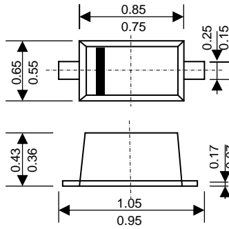
SOD-923
