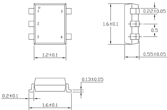
SOT-553
