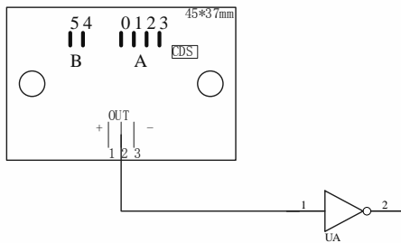
二：电平信号示意图
