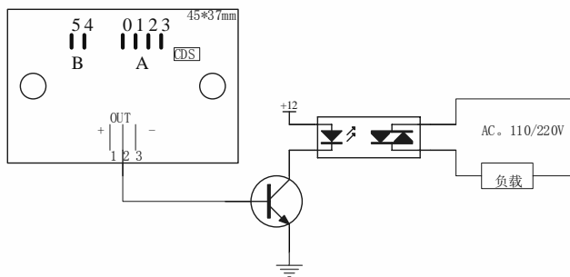
四：交流负载线路图
