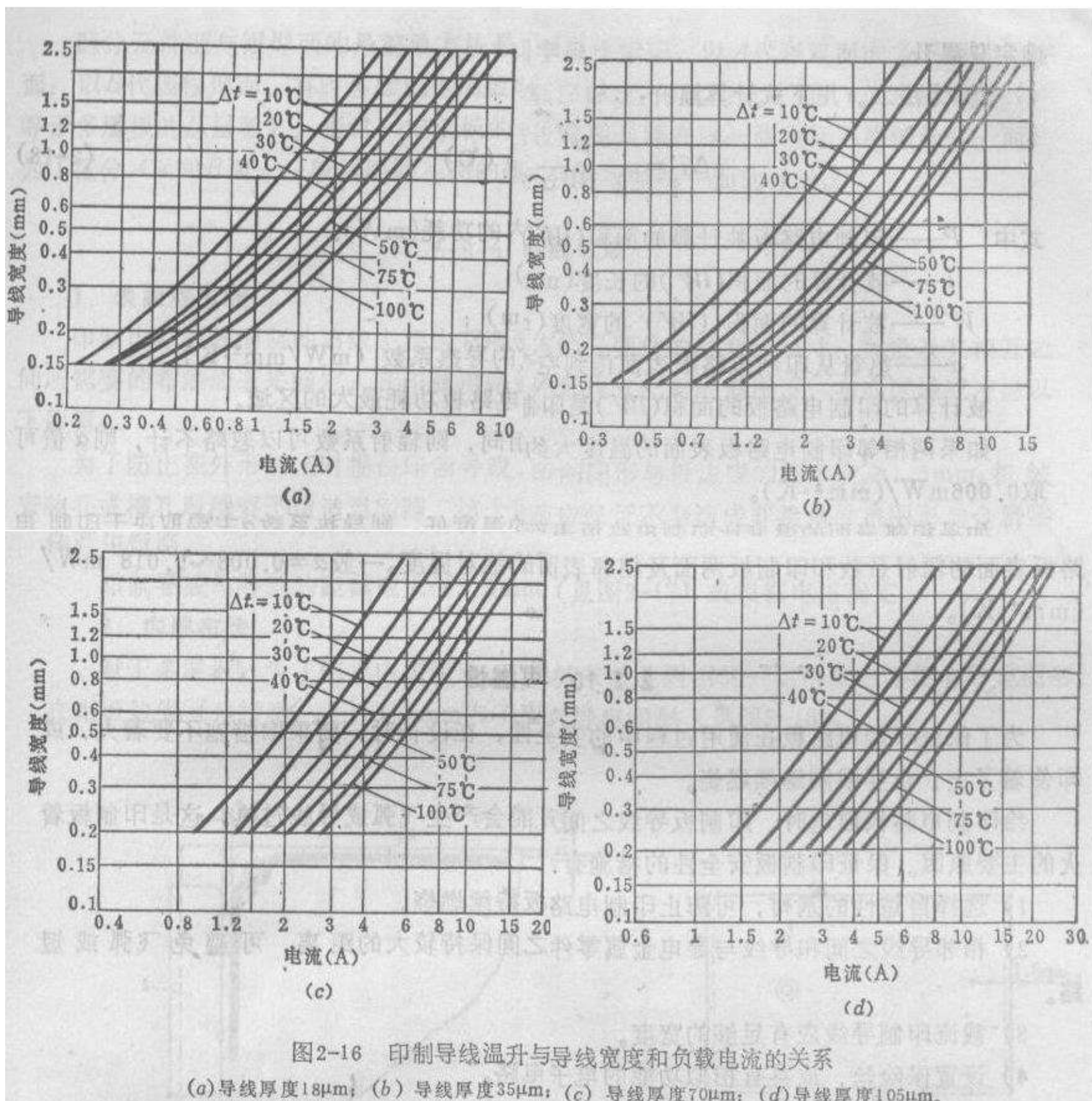
走线宽度/电流关系对照表【jpg】2003781246352838.jpg(158K)(xlander)
