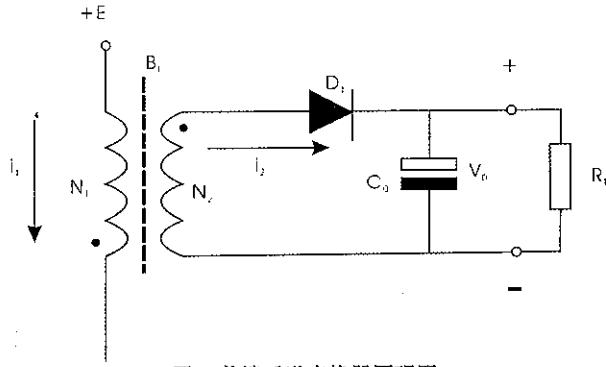
图1 单端反激变换器原理图
