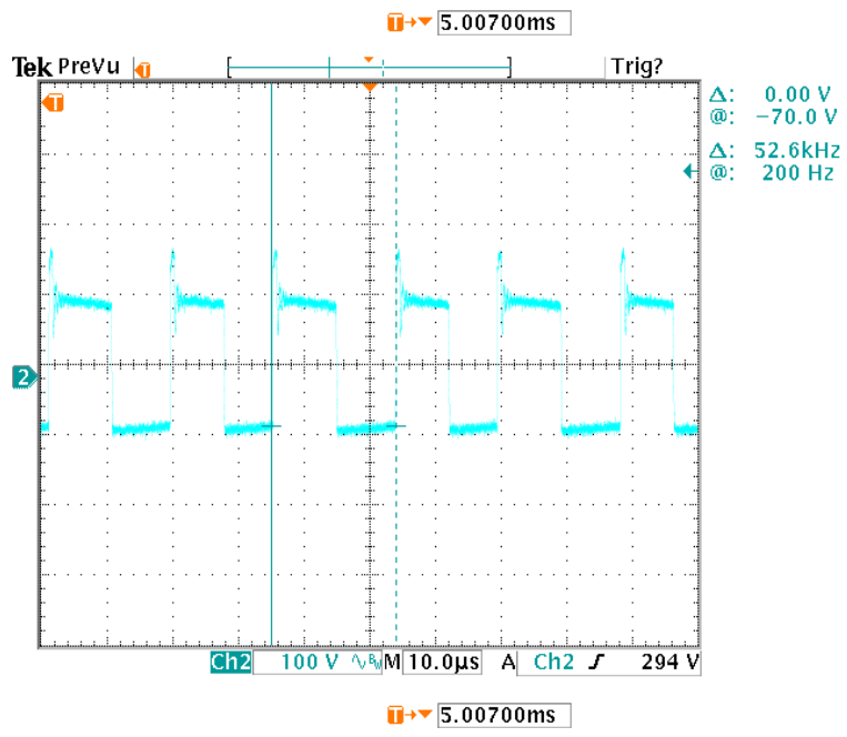
0.5A 时波形
