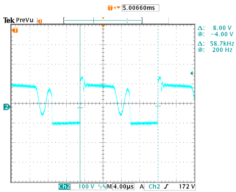
空载波形
