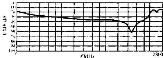
图 18 有中心线的共模扼流圈的典型响应曲线
