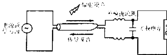
图8 差模噪声的抑制
