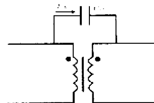
图 12 变压器初级和次级绕组之间的耦合电容
