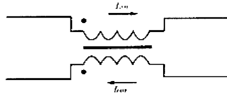
图 13 理想共模扼流圈中的差模信号
