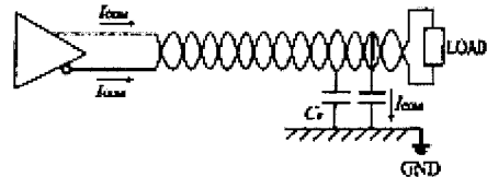
图6 无屏蔽对绞线系统中的共模信号
