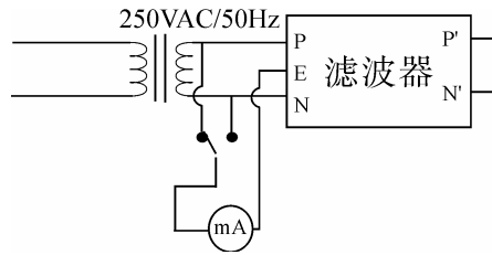
泄漏电流测试电路
