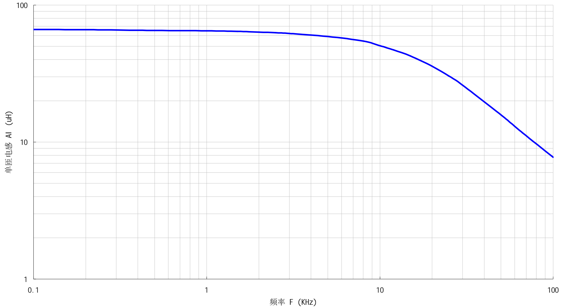
GR2008 频率特性曲线图
