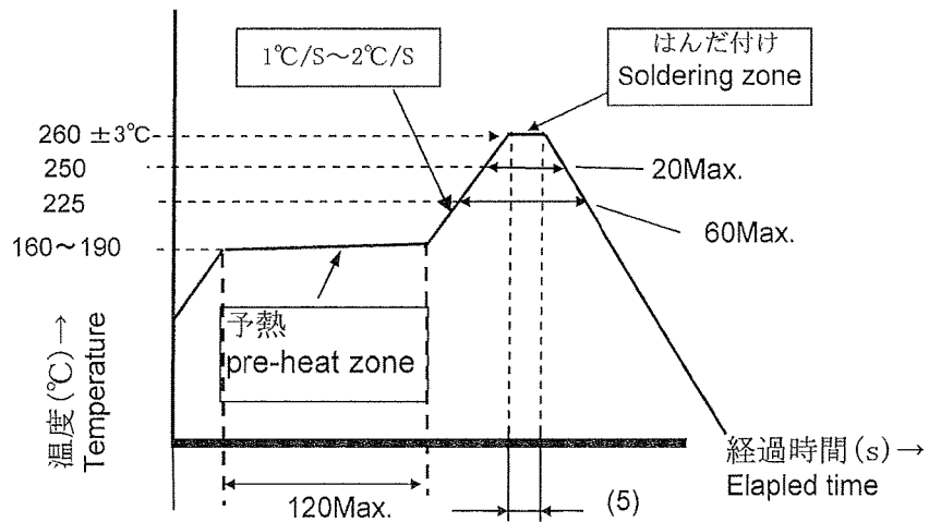
部品耐熱性評価用温度プロファイル (本体表面温度) Temperature profile for evaluation of solder heat resistance (a component's surface)
