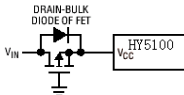
图 6：低损耗输入反向极性保护
