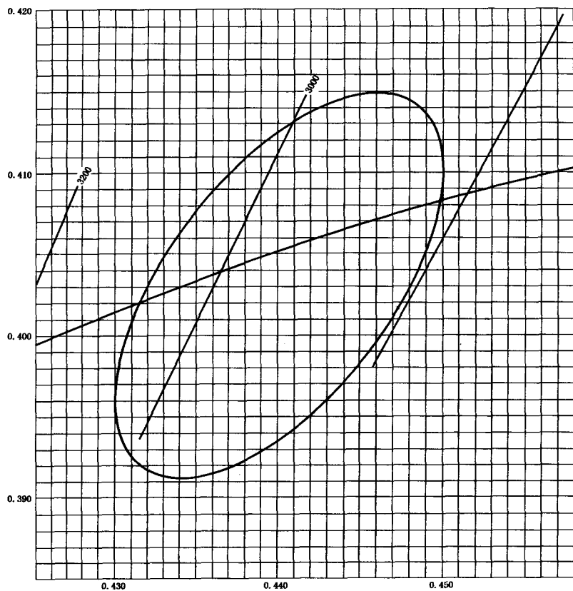
图 D5 标准暖白色的容差范围
