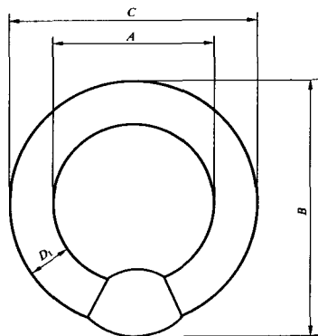
图 5 环形荧光灯尺寸定位图
