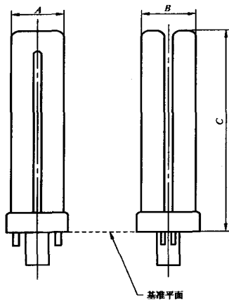
图 2 四管类单端荧光灯尺寸定位图
