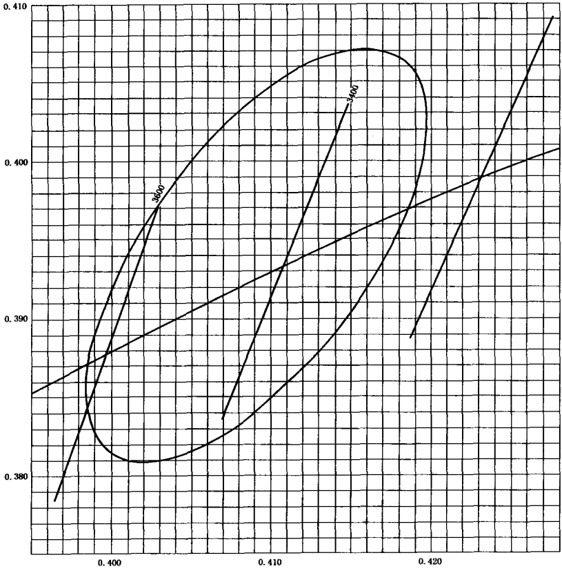
目标值 x=0.409, y=0.394 图 D4 标准白色的容差范围
