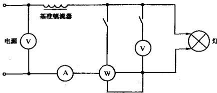
图 B2 内启动灯光电特性测量用电路图
