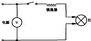
图 A1 内启动灯试验电路图
