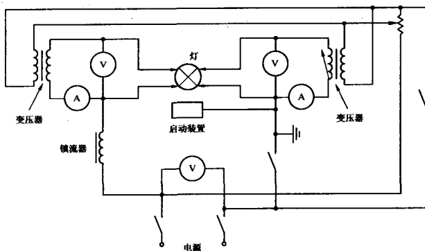
图 A3 无外接启动器电路的灯启动试验电路图
