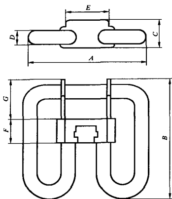
图 4 方形单端荧光灯尺寸定位图
