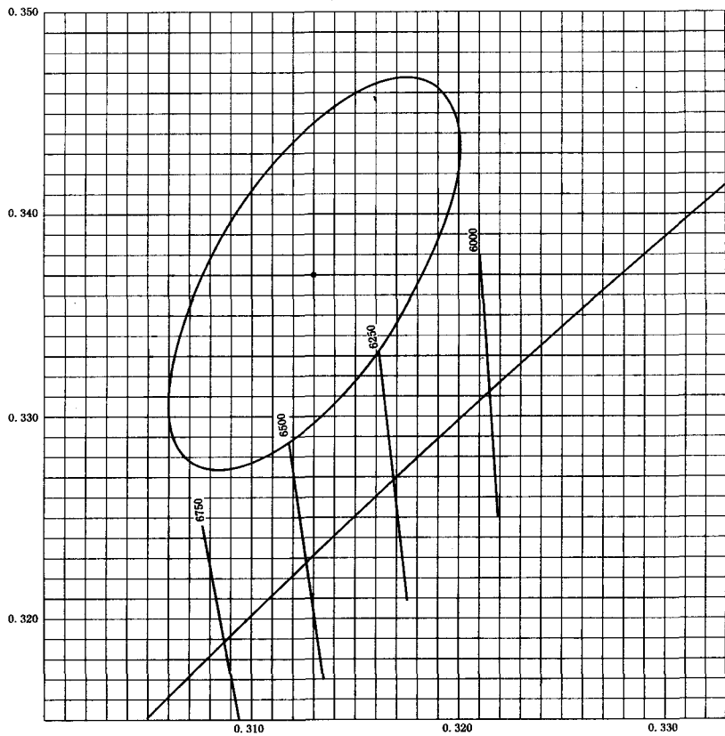
目标值 x=0.313, y=0.337 图 D1 标准日光色的容差范围
