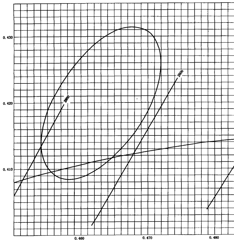
图 D6 标准白炽灯色的容差范围
