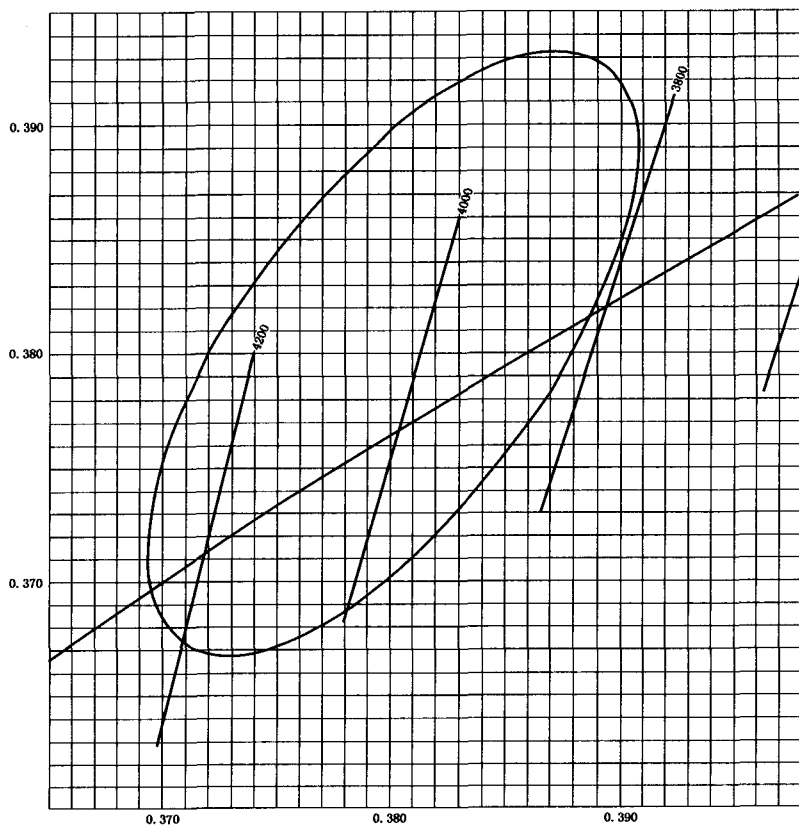
图 D3 标准冷白色的容差范围
