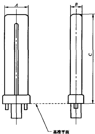
图 1 双管类单端荧光灯的尺寸定位图
