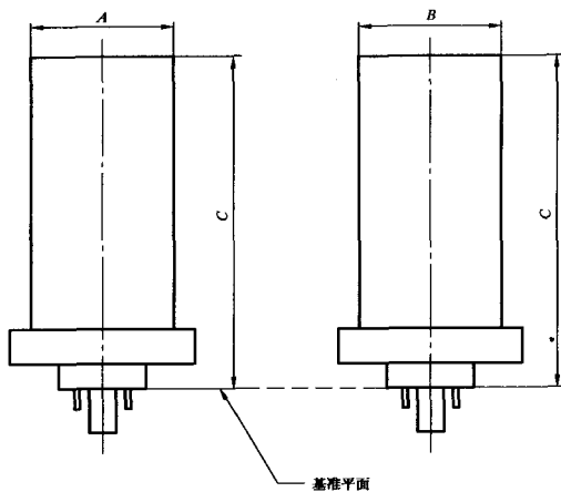
图 3 多管类单端荧光灯尺寸定位图
