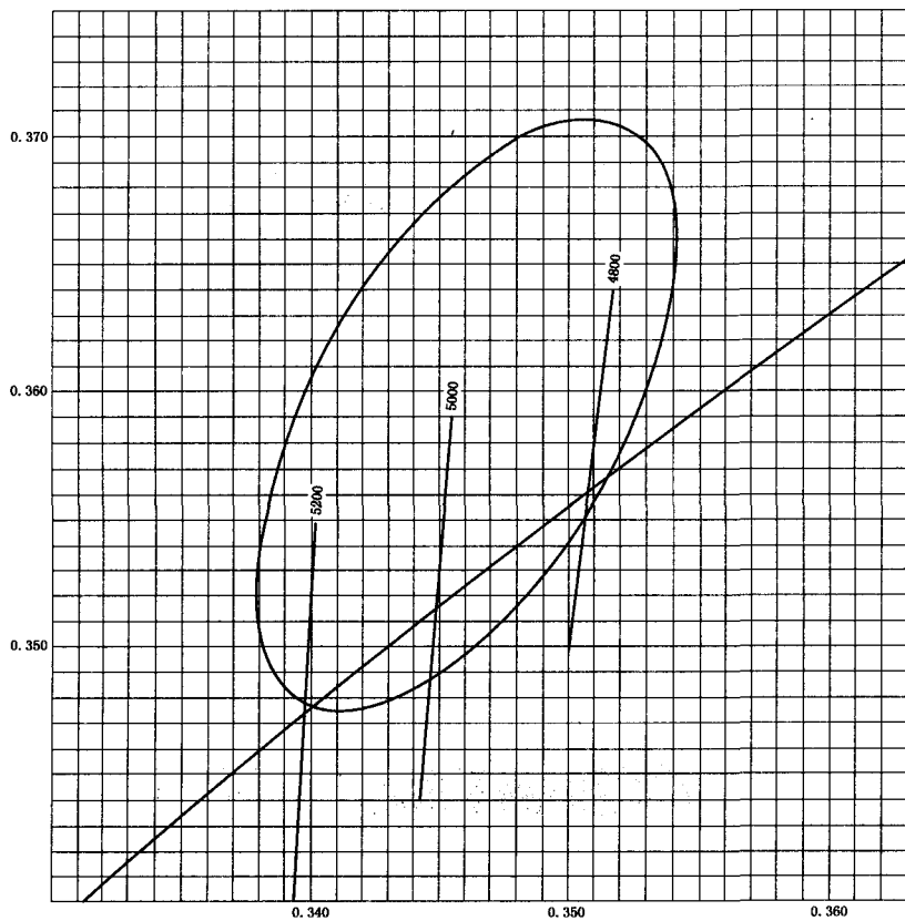
图 D2 标准中型白色的容差范围
