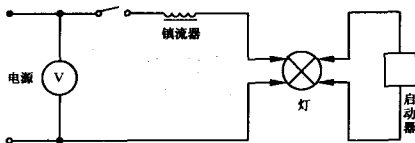
图 A2 外启动灯试验电路图
