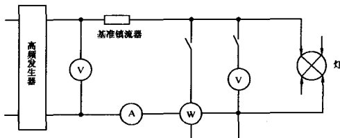
图 B4 采用高频工作的灯光电特性测试用电路图
