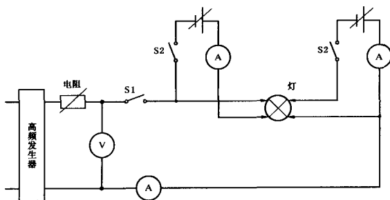
图 A4 采用高频工作的预热阴极灯试验电路图
