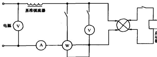
图 B3 外启动预热阴极灯光电特性测量用电路图
