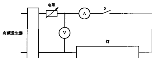
图 A4 采用高频工作的预热阴极灯启动试验用电路图
