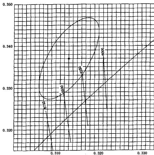
图 C1 标准色 F6500 的容差范围
