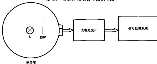
a. 积分法测量光通量示意图
