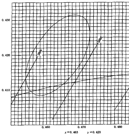
图 C6 标准色 F2700 的容差范围
