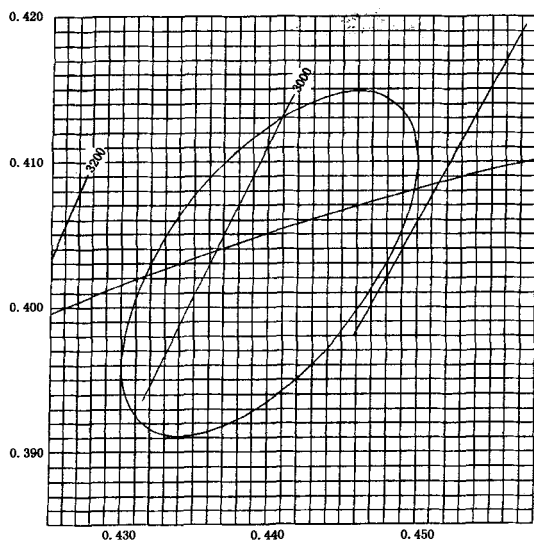
图 C5 标准色 F3000 的容差范围
