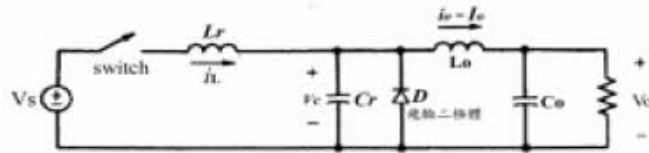
(圖 a) 零電流切換之共振式轉換器
