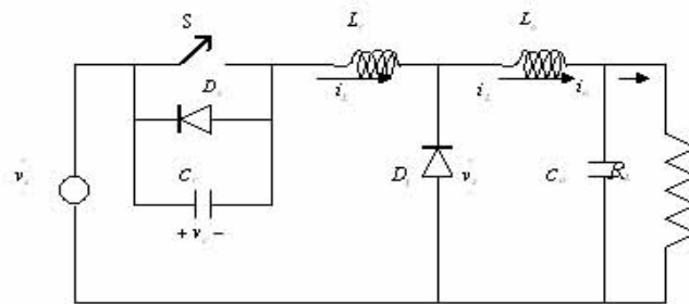
(a) 零電壓切換共振式電路圖
