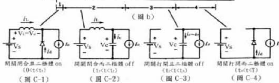
圖 1 ZCS 開關共振式直流至直流轉換器
