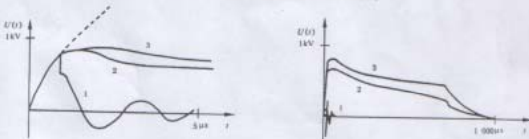
图 S2 不带电涌抑制器绝缘击穿时的波形
