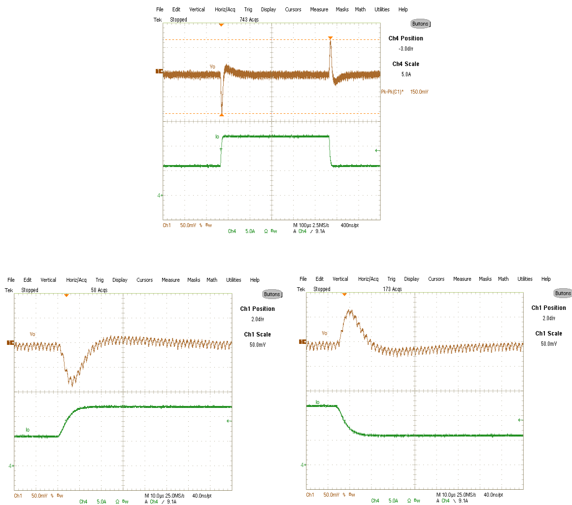
Fig. 23. Transient Response, 6A to 12A step Ch 1 : V_{out} , Ch 4 : I_{out}
