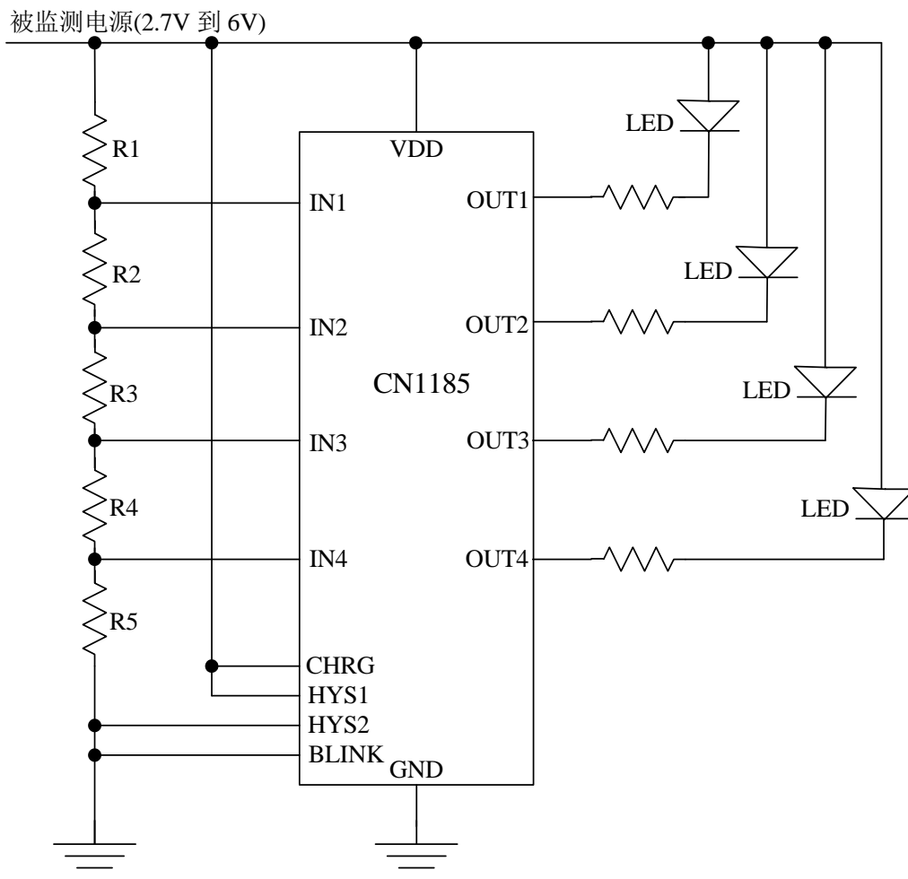
图 1 典型应用电路
