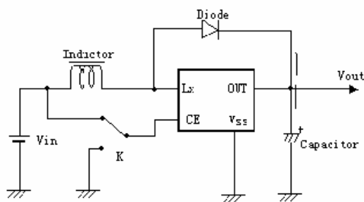
For use Chip Enable(CE)
