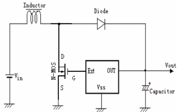
For use external transistor(N_MOS)
