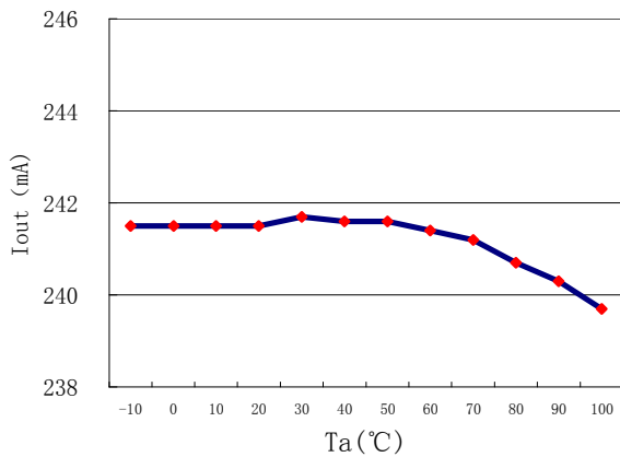
c) 环境温度对输出电流曲线图
