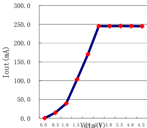
a) Vdim 对输出电流曲线图
