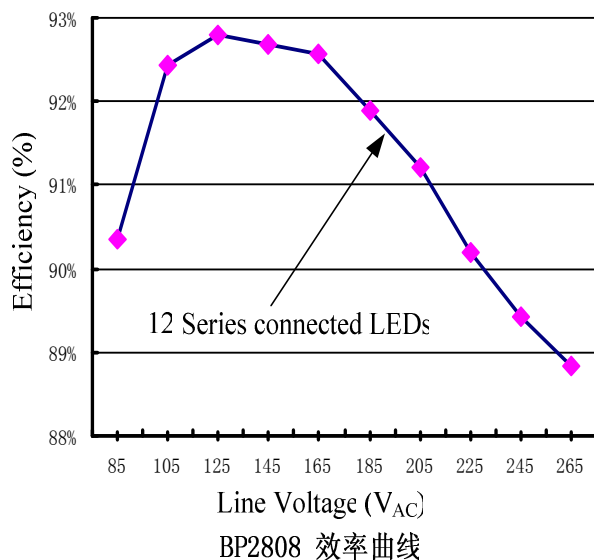
图表 1 效率和恒流特性
