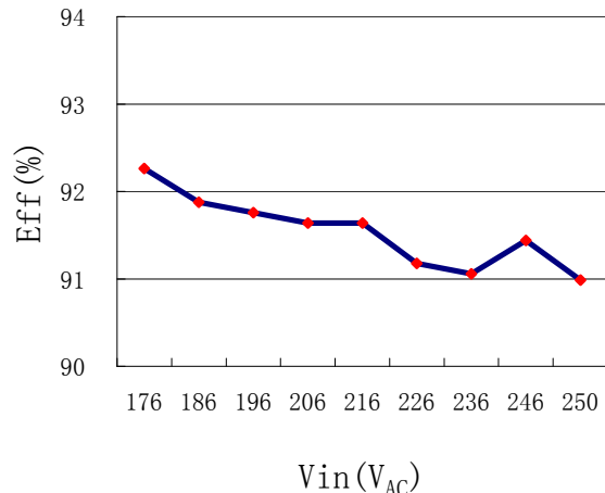
d) 输入电压对系统效率曲线图
