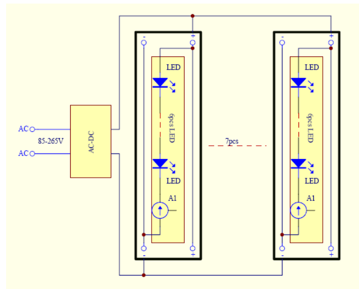
LED电源标准化设计路线
