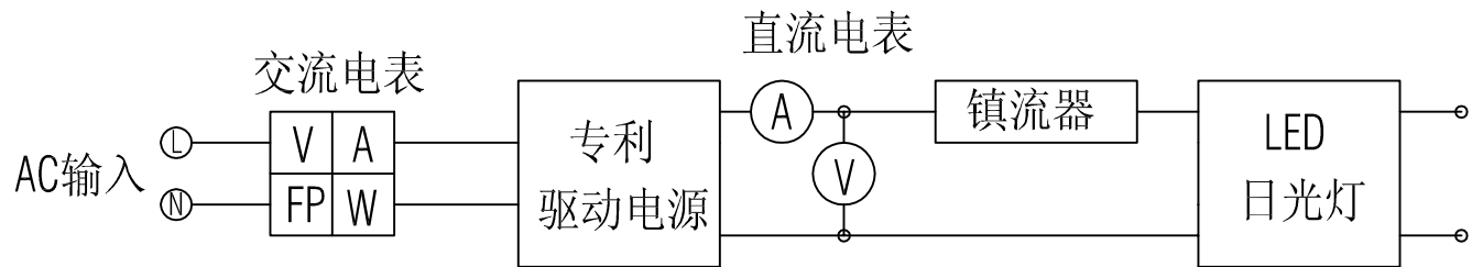
单端带镇流器供电测试接线图
