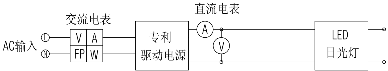
单端无镇流器供电测试接线图
