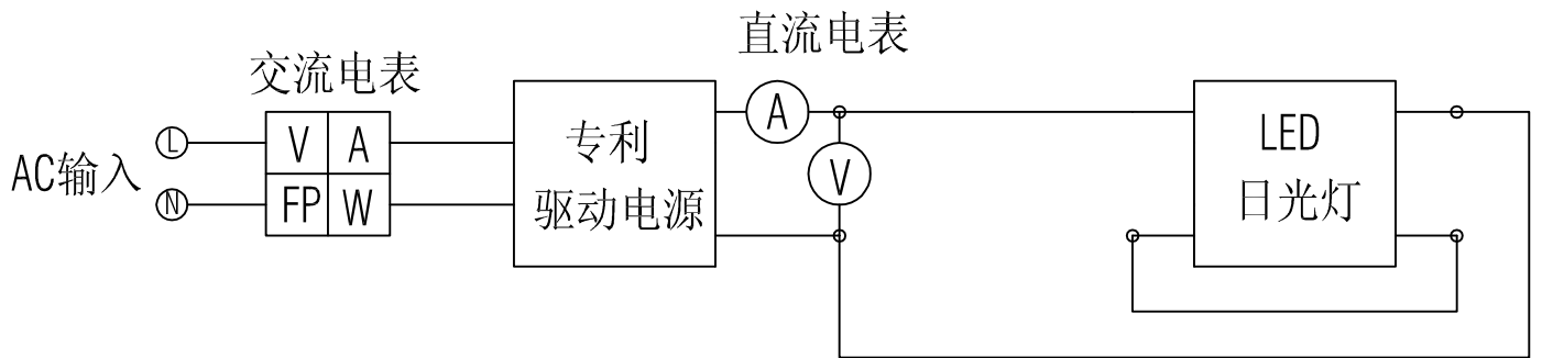
双端无镇流器供电测试接线图
