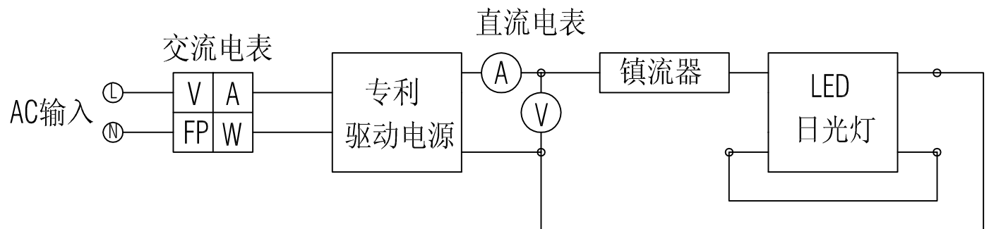
双端带镇流器供电测试接线图
