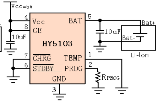
适合既不需要充电状态指示，也不需要电池温度监测功能的应用
