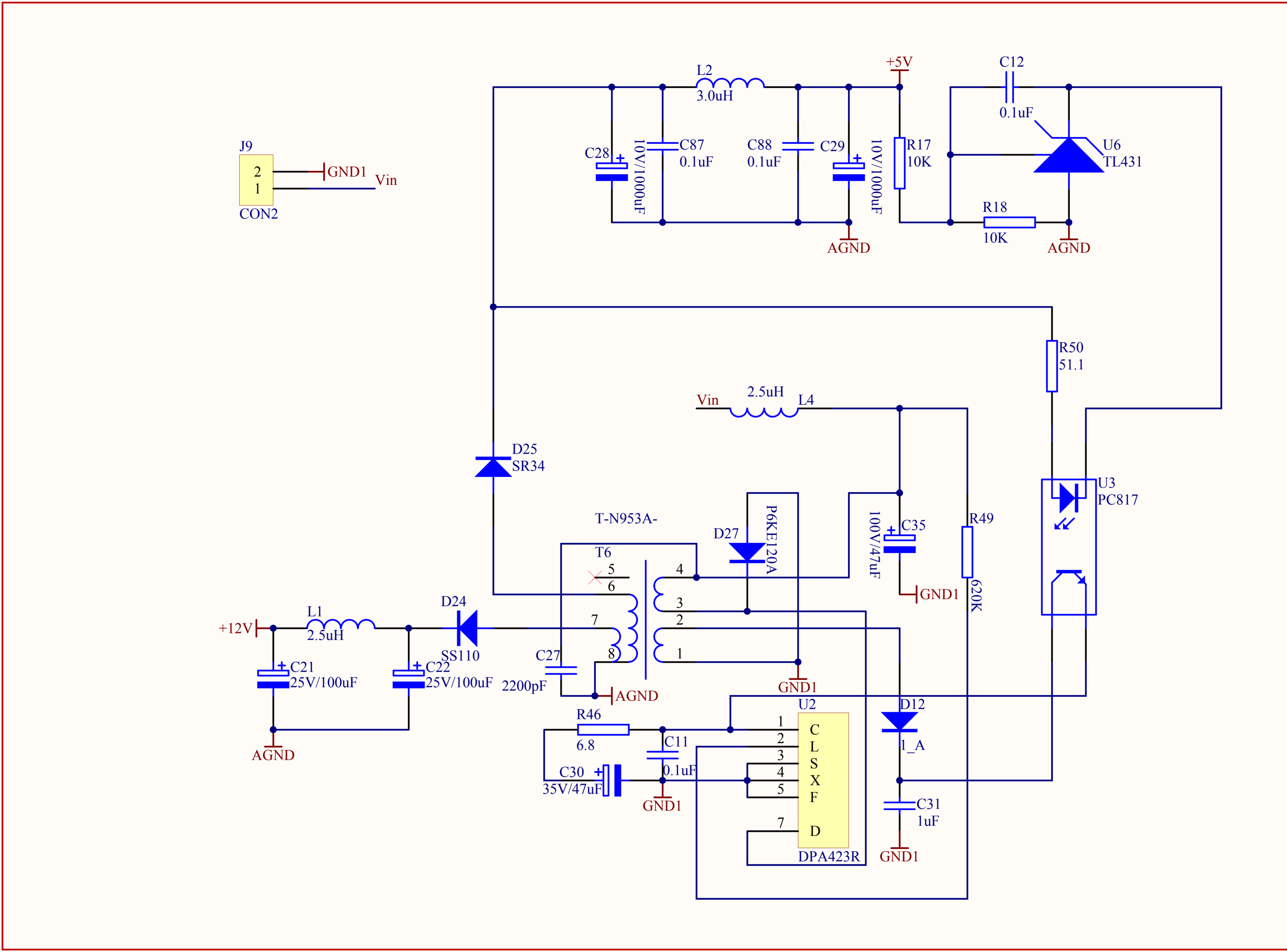
内部交直流供电电路
