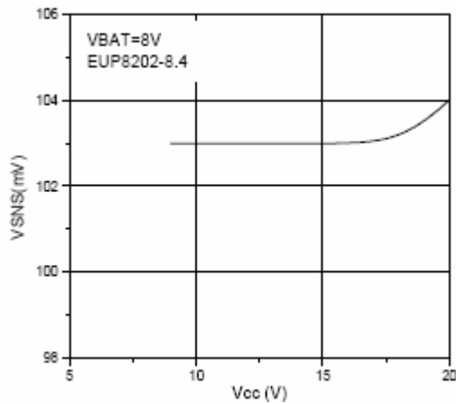
电流模式检测电压 ( V_{SNS} ) 与电源电压 ( V_{CC} )
