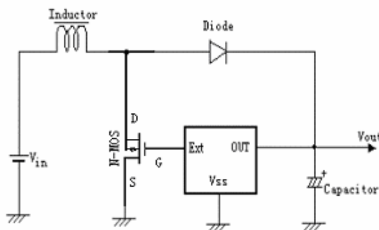
扩型产品使用示意图
