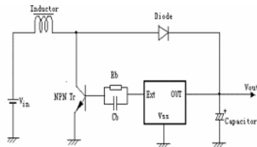
扩型产品使用示意图
