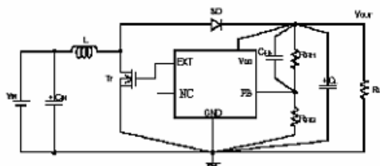
可调扩型产品使用示意图
