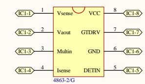
IC旁路电路
