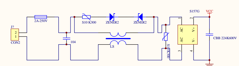
输入电路
