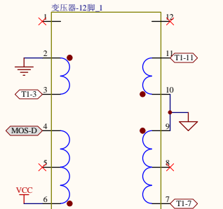
变压器
