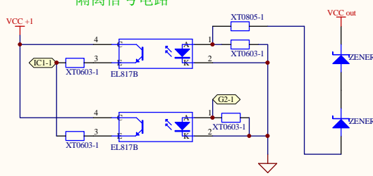
隔离信号电路
