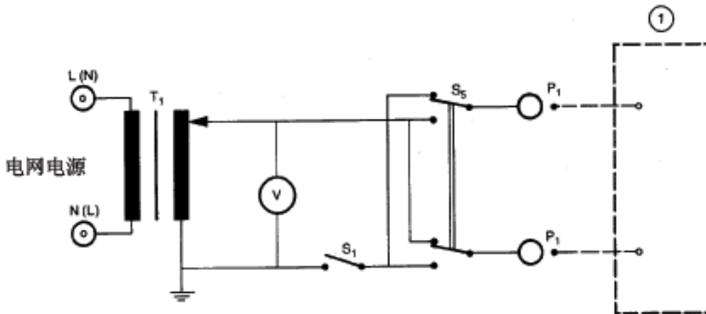
图10 供电网的一端近似地电位时的测量供电电路(19.4b))
