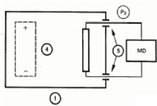
图 27 内部电源供电设备的患者辅助电流的测量电路(见 19.4j)
