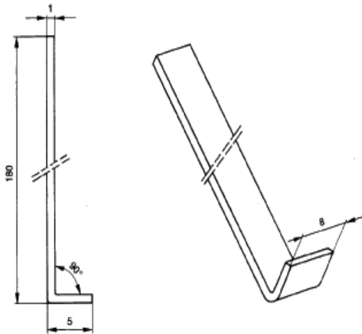
尺寸单位为毫米 材料：钢 图9 试验钩(见第16章)
