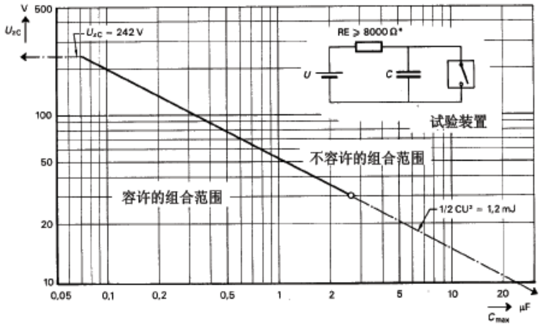
图 30 在乙醚蒸气和空气混合成的最易燃气体中电容电路上测得的最大容许电压 U_{zC} 和电容 C_{max} 的函数关系(见 40.3)
