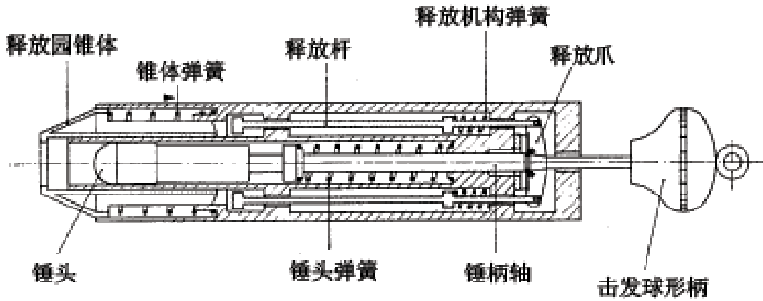
图 G1 冲击试验装置 (见第 21 章)
