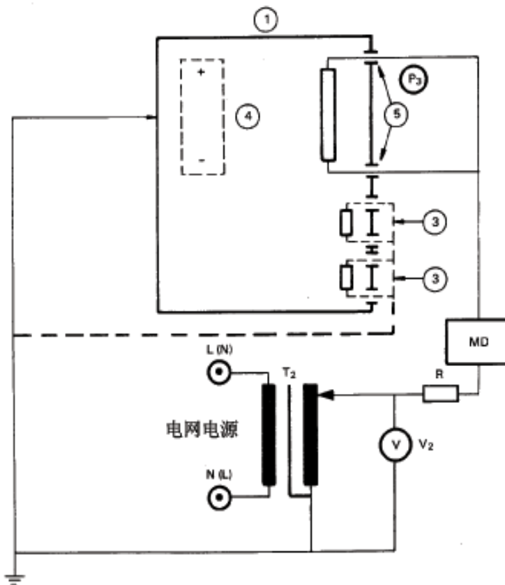
图 24 内部电源供电设备从 F 型应用部分至外壳的患者漏电流的测量电路(见 19.4h))
