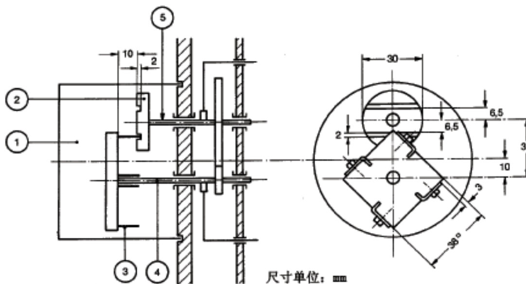
图 F1 试验装置
