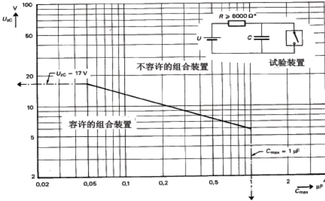
图 33 在乙醚蒸气和氧混合成的最易燃气体中电容电路上测得的最大容许电压 U_{zc} 和电容 C_{max} 的函数关系(见 41.3)
