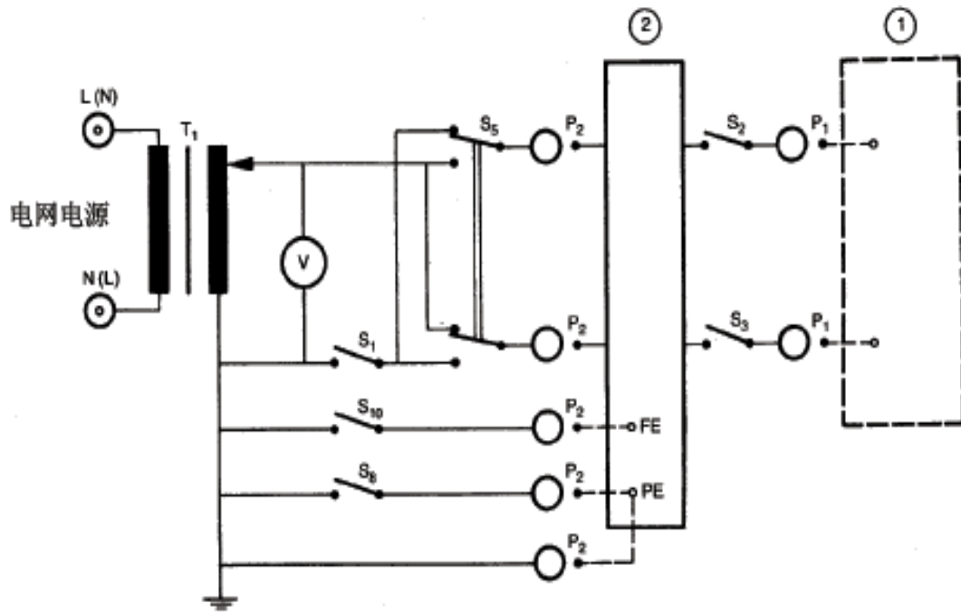
图 14 由规定按 I 类或 II 类单相电源供电的设备的测量供电电路 在 I 类时，不使用保护接地连接和 S_8 (19.4b)
