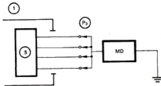
带 B 型应用部分的设备 从连在一起的所有患者连接线测 说明见 87 页
