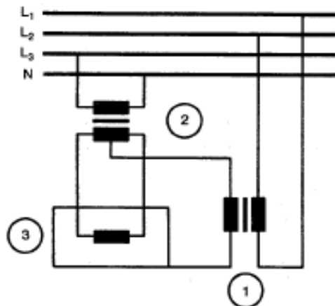
图 28 电热元件在工作温度下电介质强度试验电路图例(见 20.4)
