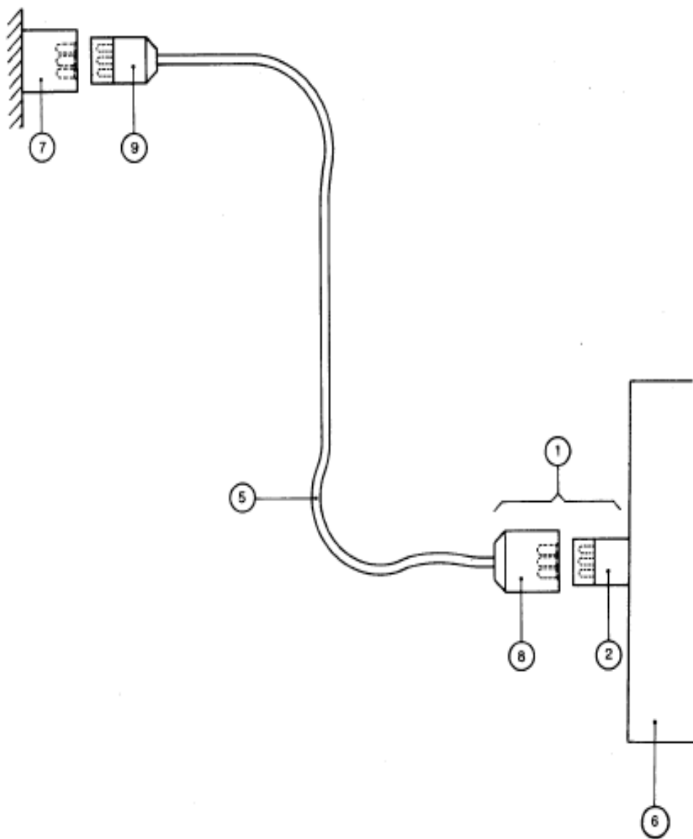
1-设备连接装置；2-设备电源输入插口；5-可拆卸电源软电线；6-设备；7-固定的网电源插座； 8-网电源连接器；9-网电源插头
