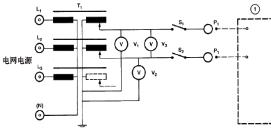
图 13 规定接至多相供电网的单相设备的测量供电电路(19.4b)
