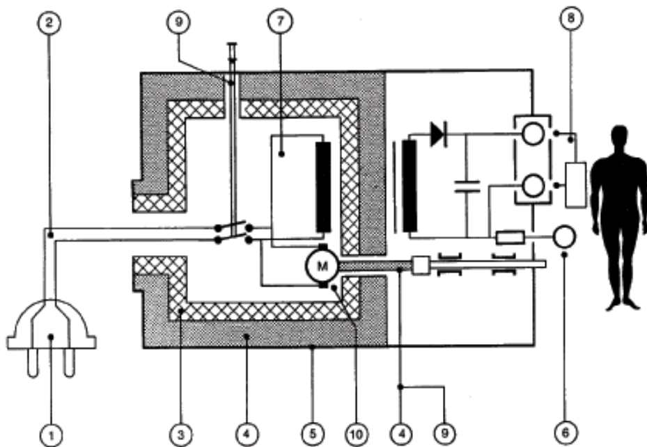
-网电源插头； -电源软电线； -基本绝缘； -辅助绝缘； -外壳； -功能接地端子； -网电源部分； -应用部分； -加强绝缘； -有可触及轴的电动机
