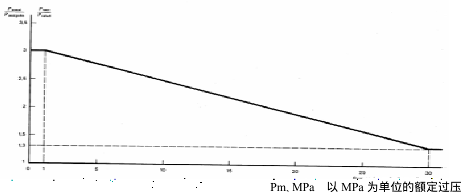
图 38 水压试验压力与最高容许工作压力的比例关系
