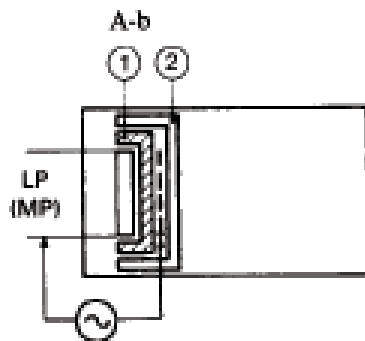
-- 基本绝缘； -- 辅助绝缘
