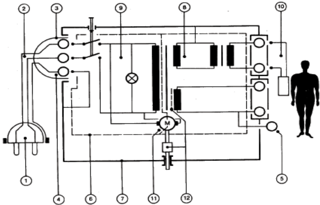
-护接地接点的插头； -可拆卸电源软电线； -设备连接装置； -保护接地用接点和插脚； -功能接地端子； -基本绝缘； -外壳； -中间电路； -网电源部分； -应用部分； 11-有可触及轴的电动机； 12-辅助绝缘或保护接地屏蔽
