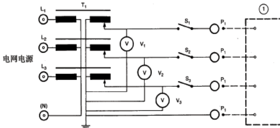
图 12 规定接至多相供电网的多相设备的测量供电电路(19.4b)
