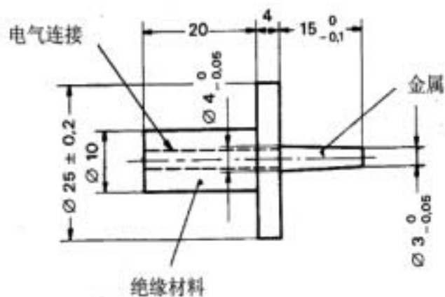
图 8 试验针(见第 16 章)
