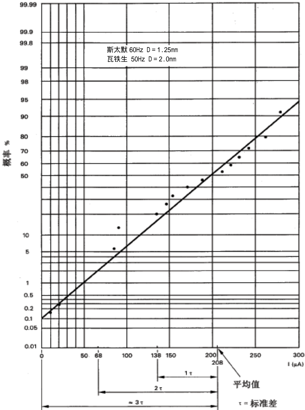
图 A1 室颤概率
