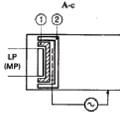
-- 基本绝缘 ; -- 辅助绝缘
