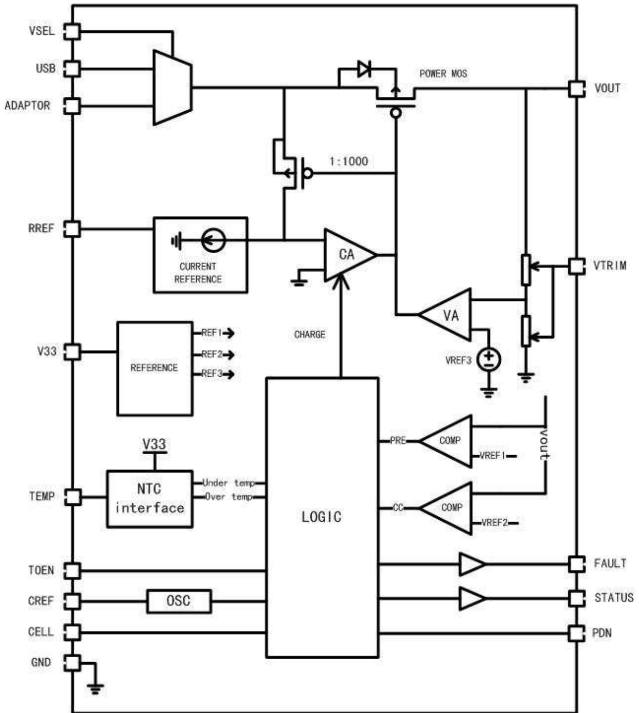
图 3. 1、HB6292 功能框图
