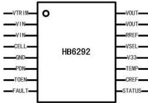
图 4.1、HB6292 管脚分布
