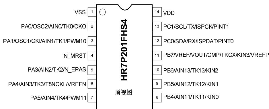
图 1-3 HR7P201 (SOP14) 顶视图
