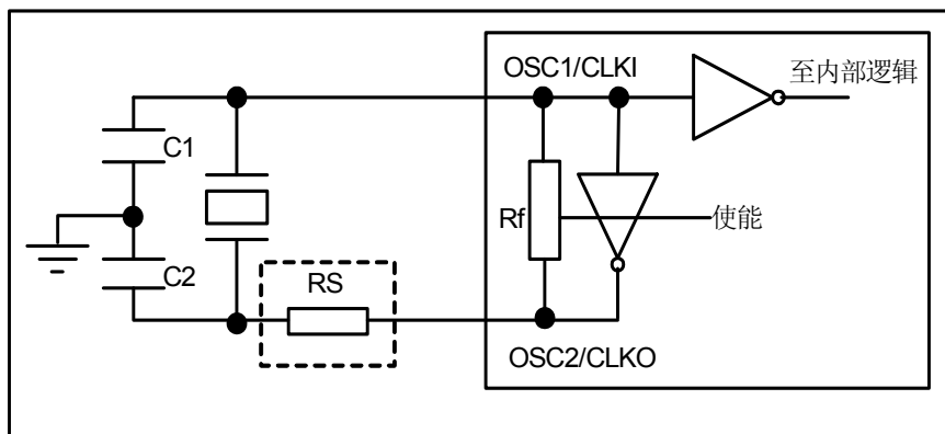
图 6-2 晶体/陶瓷振荡器模式（HS、XT）
