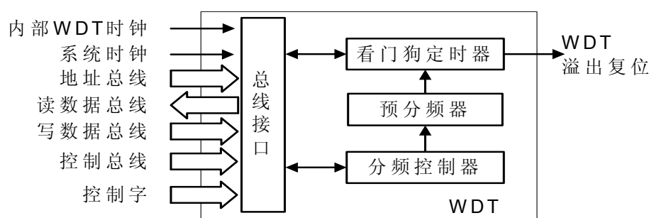
图 6-3 看门狗定时器内部结构图
