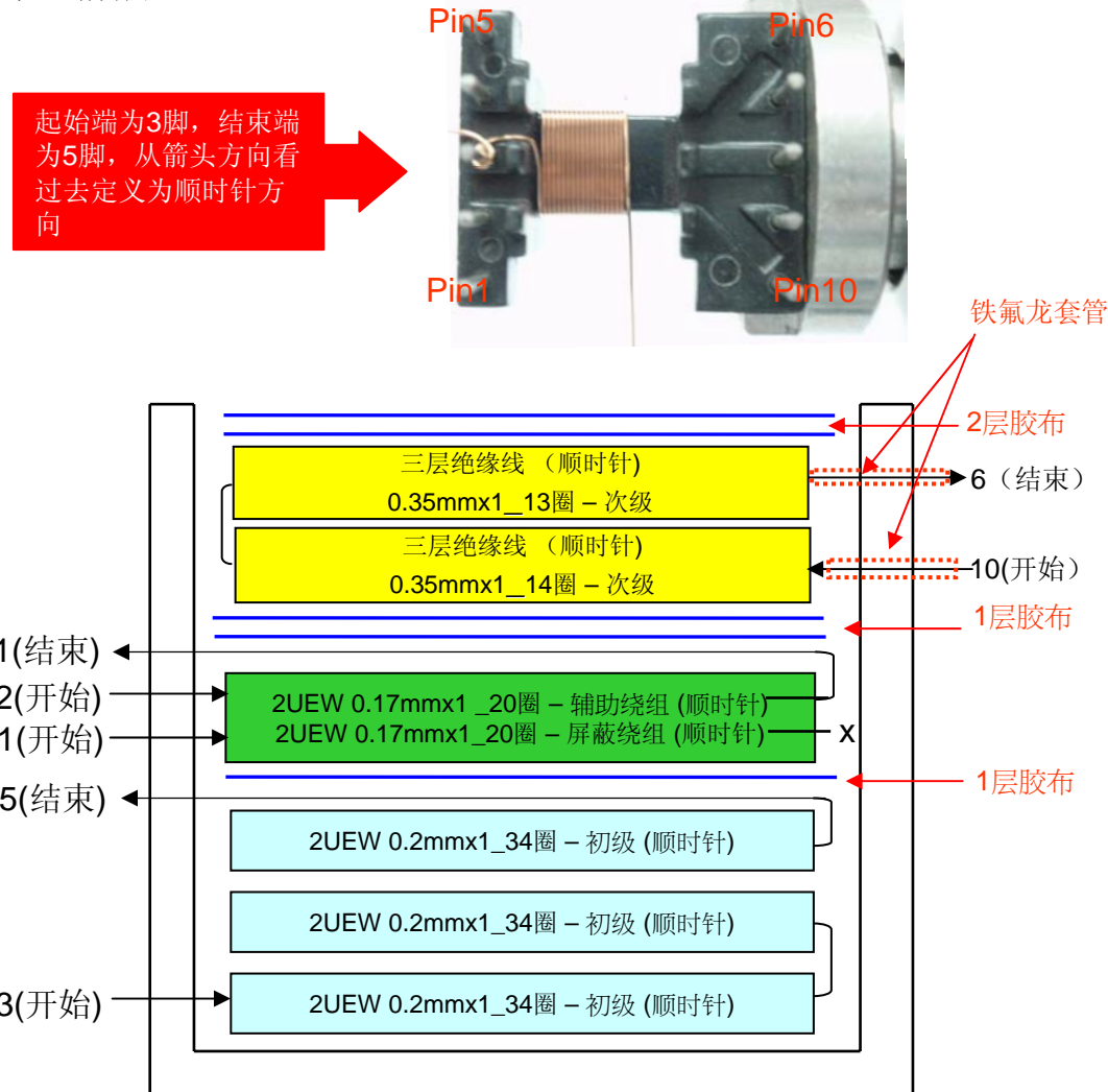
绕组结构图...
