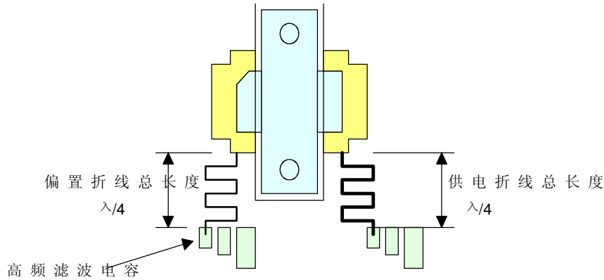
图12: 功放管偏置布线
