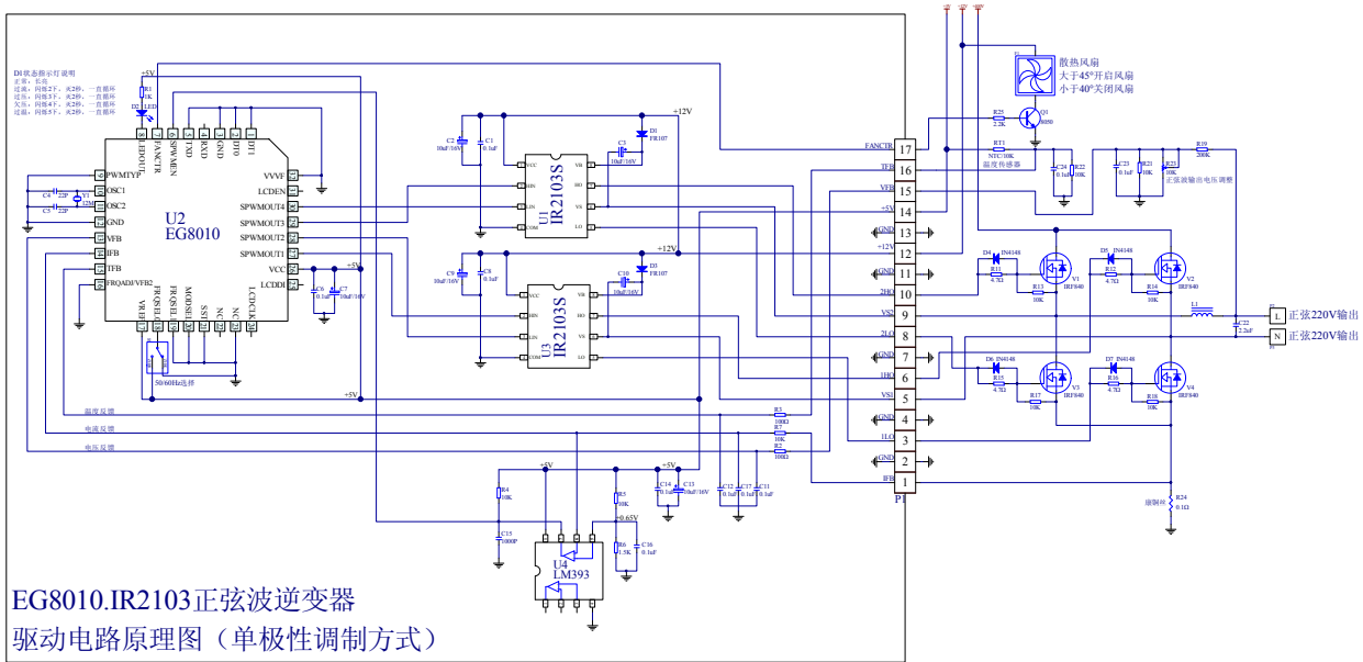
图 6-2. EG8010+IR2103S 纯正弦波逆变器典型应用电路图 (单极性调制方式)
