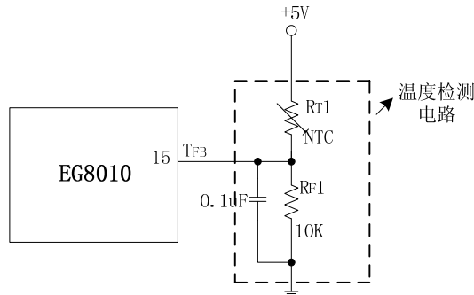
图 8.3a EG8010 温度检测电路
