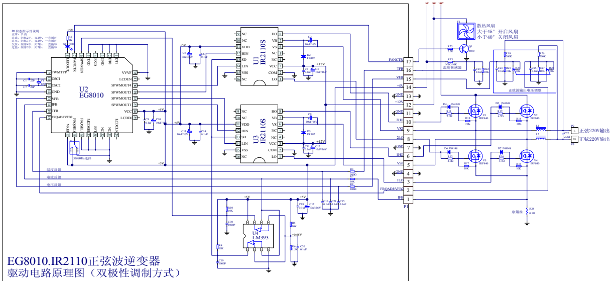
图 6-4. EG8010+IR2110S 纯正弦波逆变器典型应用电路图（双极性调制方式）
