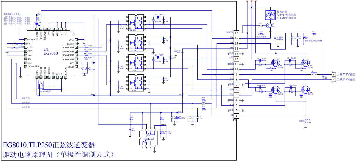
图 6-3. EG8010+TLP250 纯正弦波逆变器典型应用电路图（单极性调制方式）
