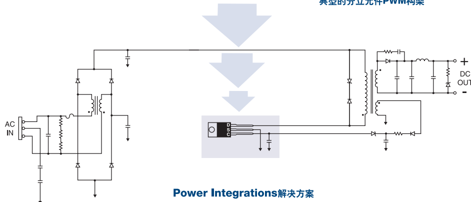
典型的分立元件PWM构架
