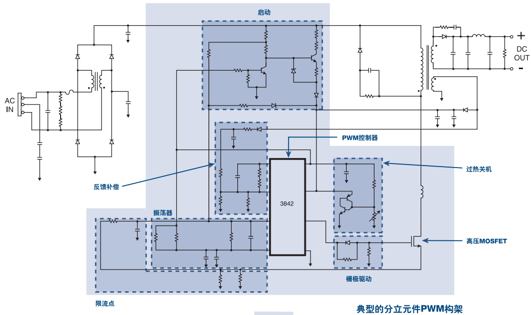
典型的分立元件PWM构架
