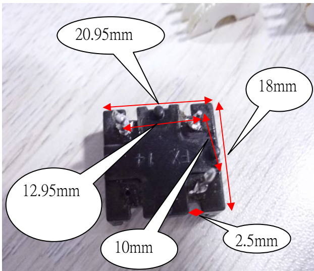
底座
