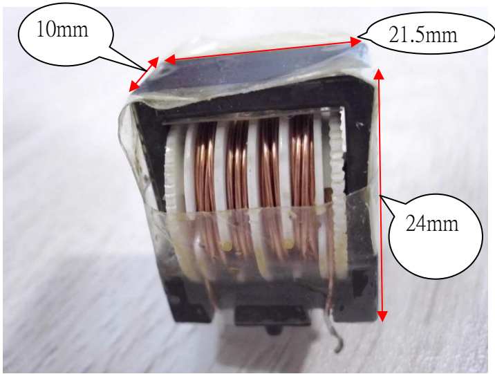
成品
