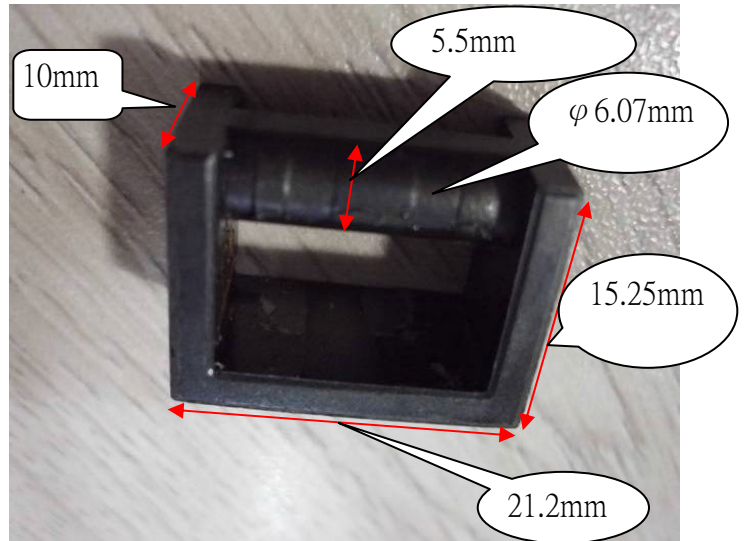
磁芯
