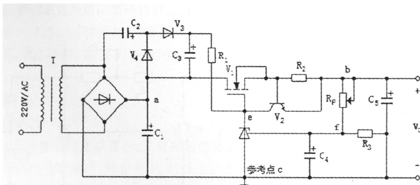
图 12 可调稳压电源
