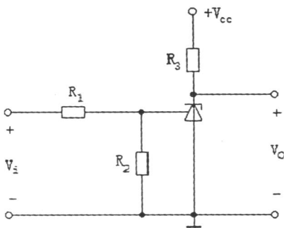
图 9 电压比较器
