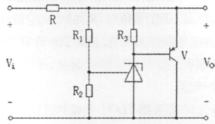
图 6 大电流基准电压源
