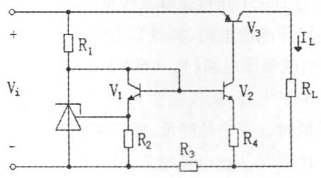
图 8 改进型恒流源电路
