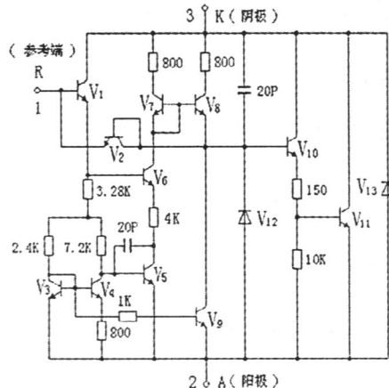
图 2 TL431 内部电路结构
