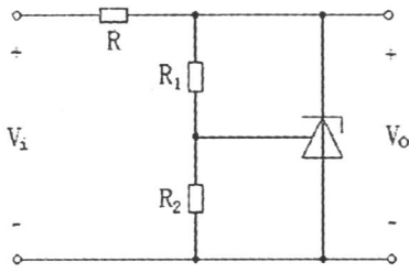
图 5 基准电压源
