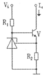
图 7 恒流源电路
