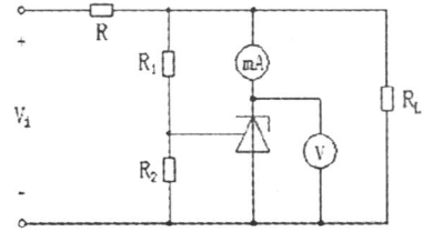
图 4 性能测试电路
