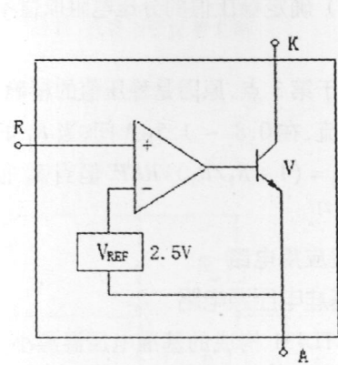
图 3 TL431 等效功能框图
