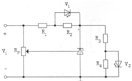
图 10 电压监视器
