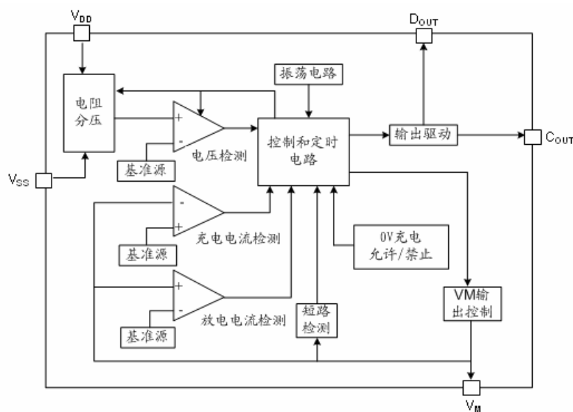
图-1 VA7028 功能框图
