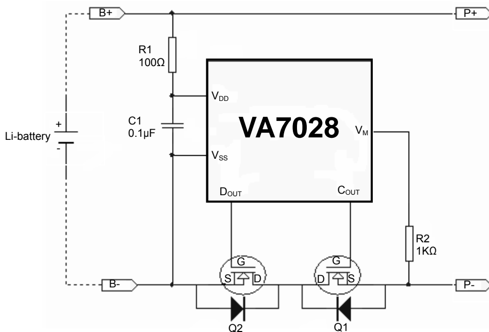
图-3 VA7028 典型应用电路图
