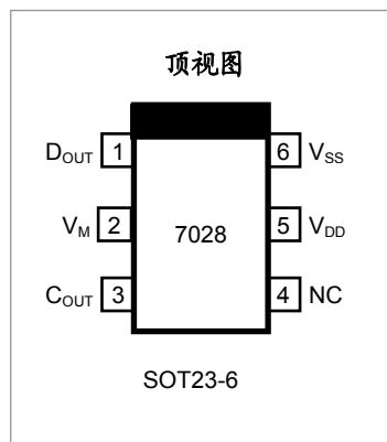
图-2 VA7028 管脚排列 (不成比例)
