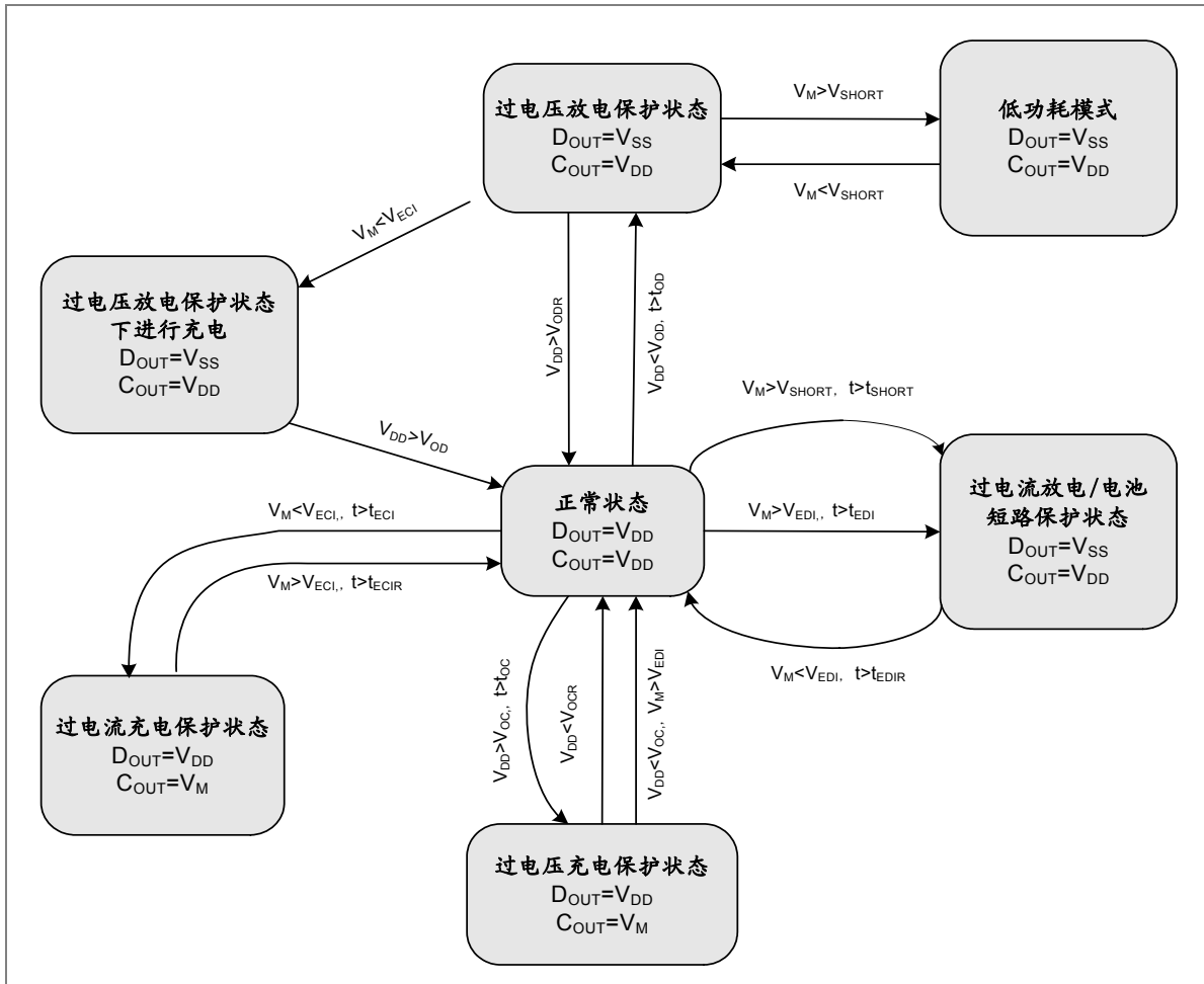
图-4 VA7028 各状态之间的转换图
