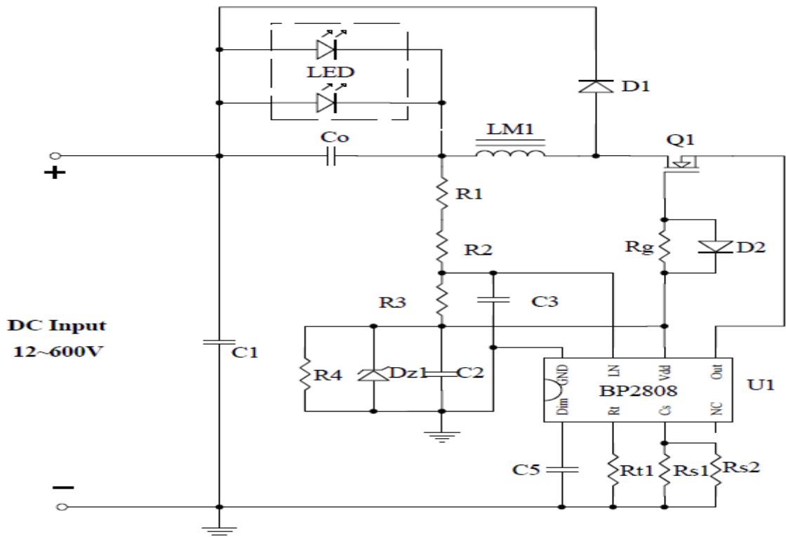
图表 2 典型应用图
