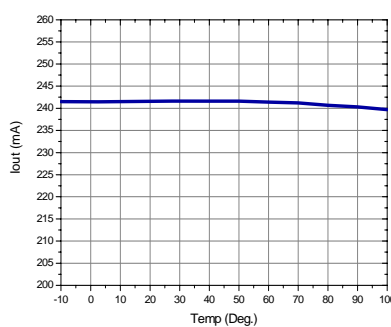
b) 输出电流vs环境温度
