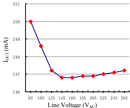
图表 1 效率和恒流特性
