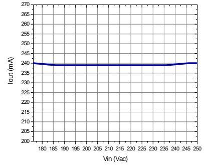
d) 输出电流 vs 输入电压
