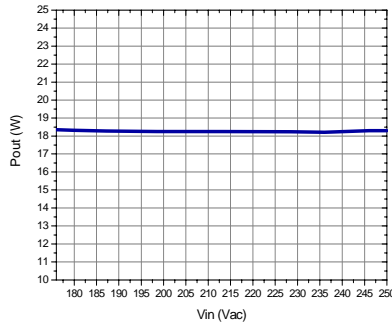
c) 输出功率 vs 输入电压
