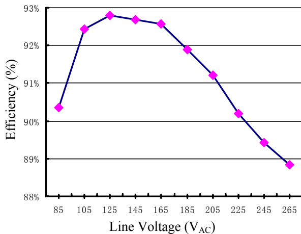
图表 1 效率和恒流特性
