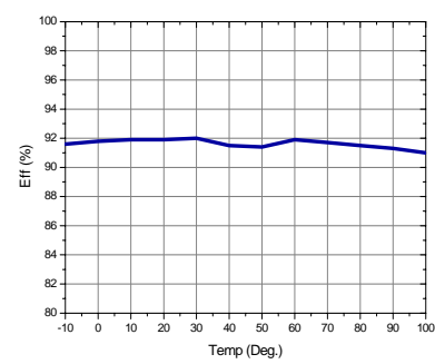
d) 系统效率vs环境温度
