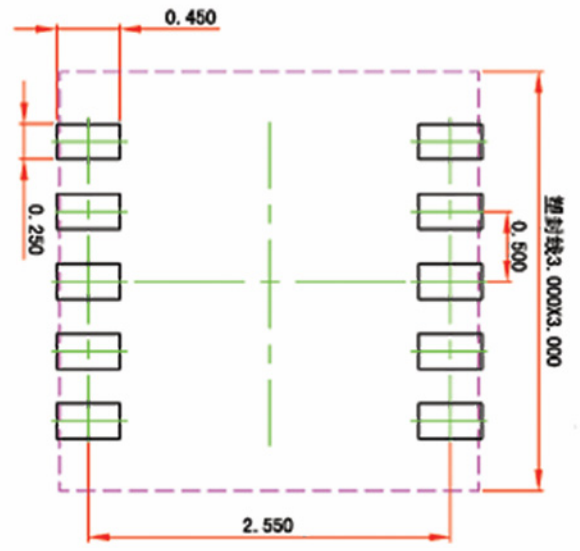
焊盘图
