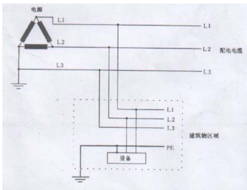
接地的相线和设备上独立的接地线
