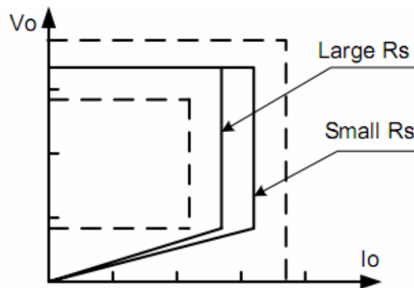
图3 改变 R_S 调节输出功率
