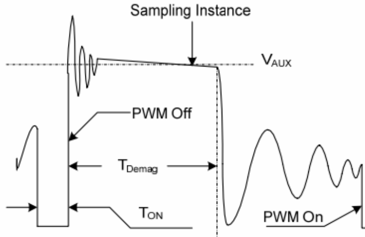
图2 辅助边电压波形
