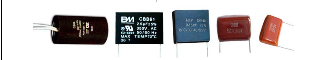
金属化聚丙烯膜电容 (CBB 电容)
