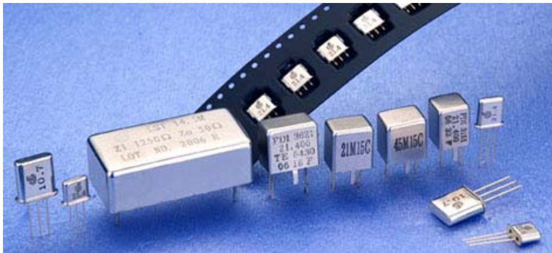
晶体滤波器
