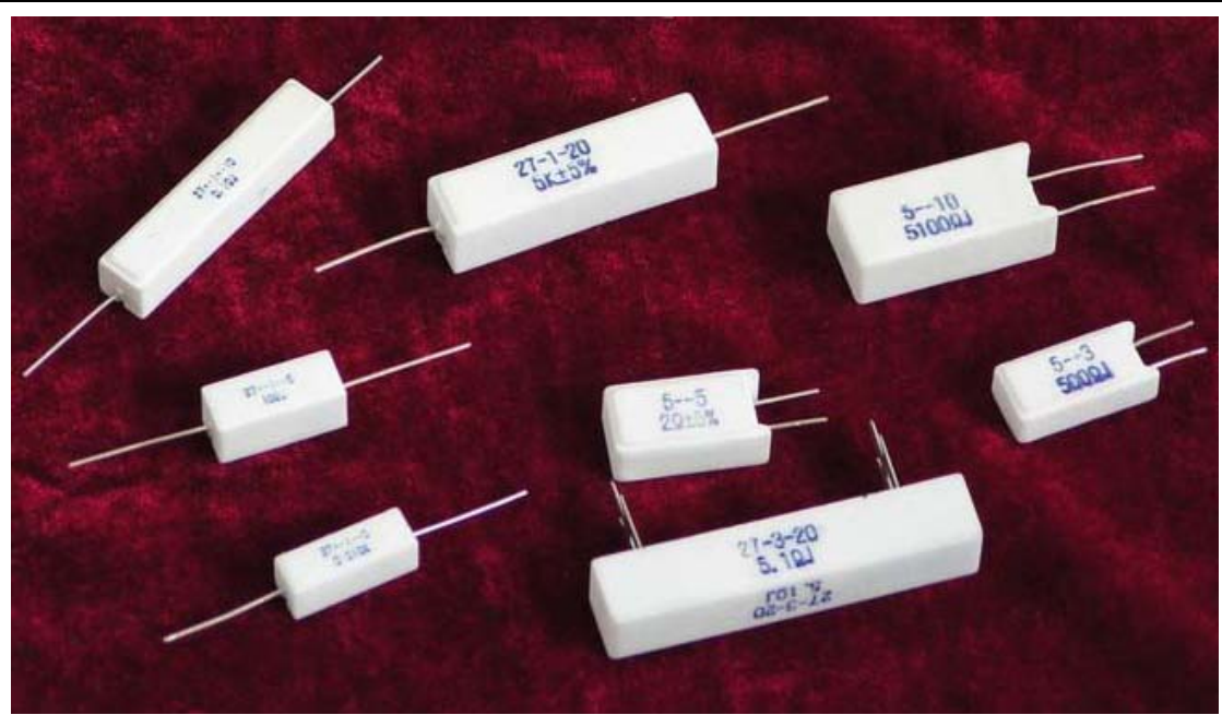
水泥电阻
