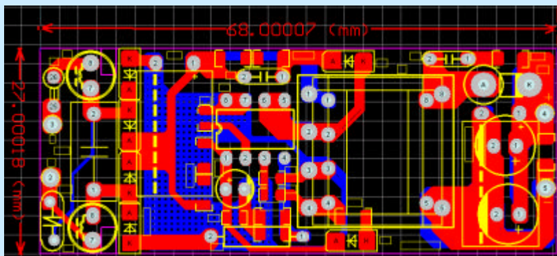
TOP层
