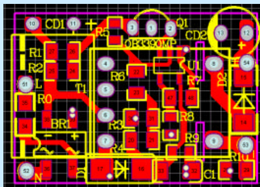
TOP层
