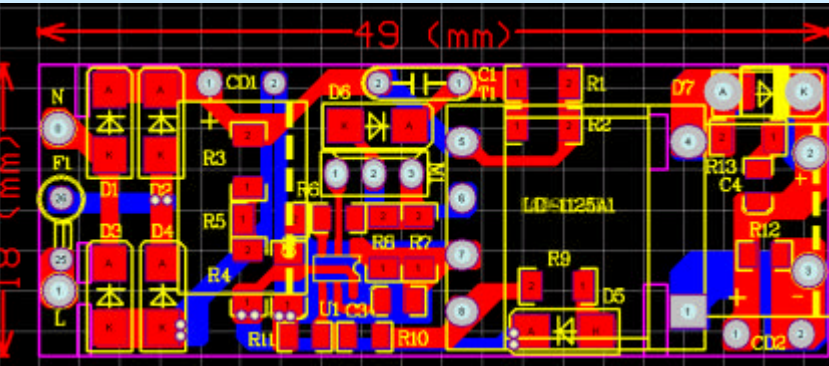
TOP层
