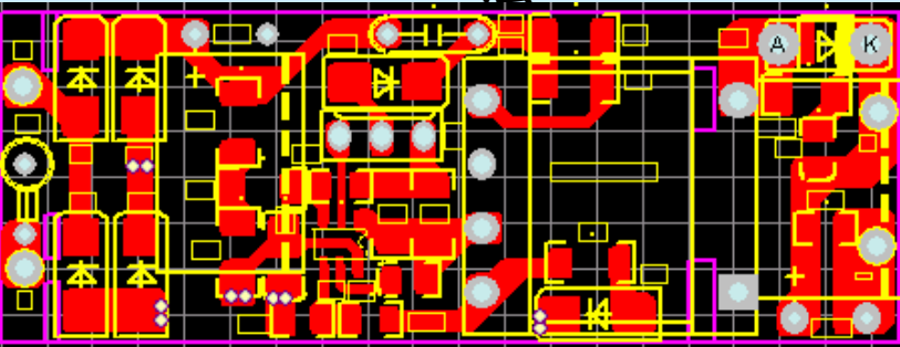
TOP层
