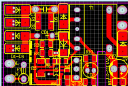
TOP层
