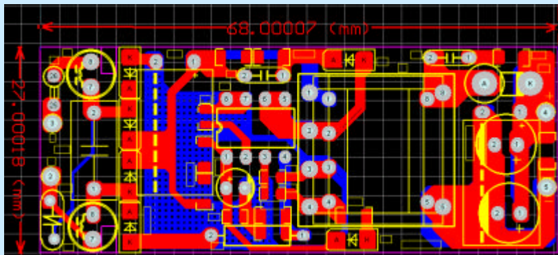
TOP层
