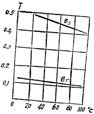
图C2 铁氧体R 2 KD B s 和B r 和温度关系
