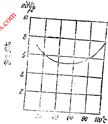
图C3 铁氧体R 2 KD损耗和温度关系
