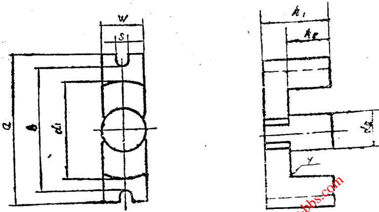
图B1 EC型磁芯
