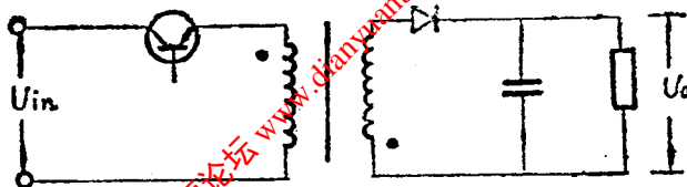
图9 单端反激式开关电源基本电路
