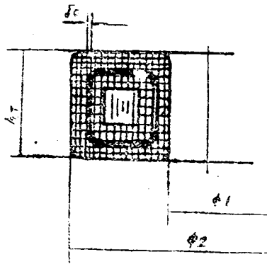
图5 环型变压器
