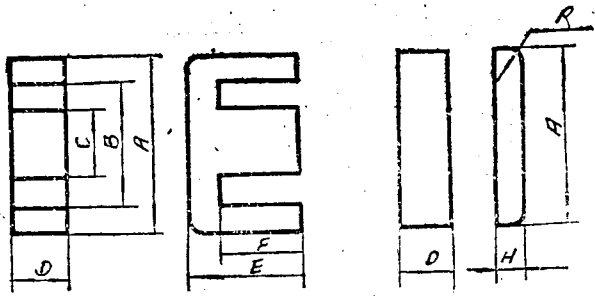
图B3 EI型磁芯
