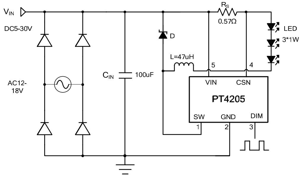
Fig1 : 3X1W application
