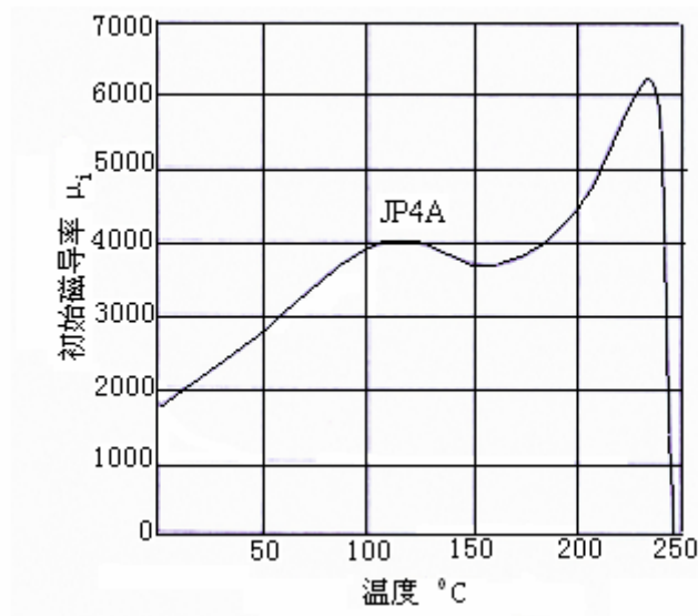
图 1 (相对)初始磁导率随温度之变化
