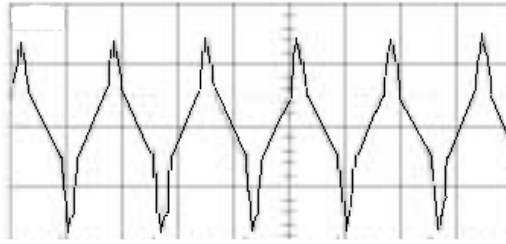
图3 电感饱和后电感线圈中的电流波形
