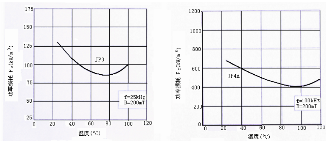
图 5 磁芯中功率损耗随温度的变化曲线
